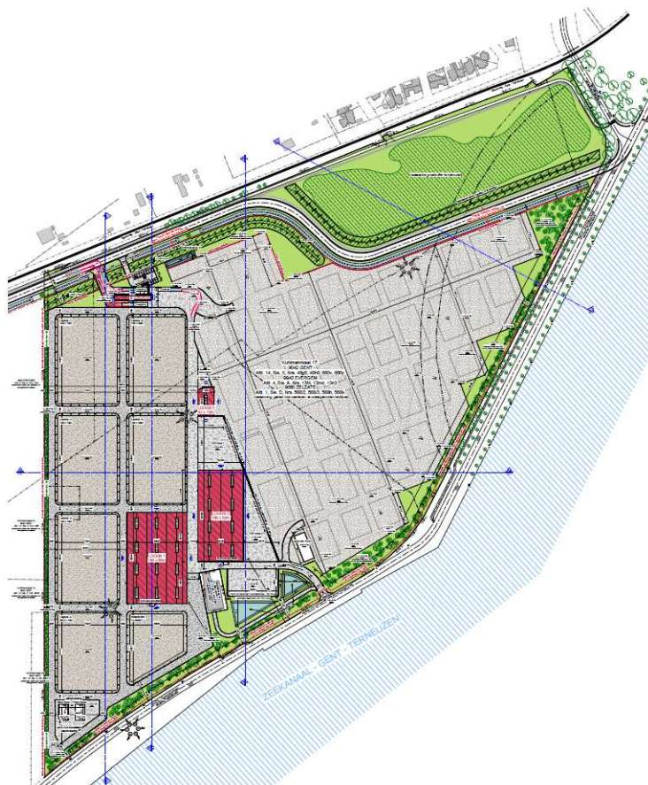
Figuur 2: Inplantingsplan
