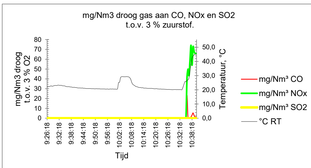
Rookgasgrafieken van Ketel 84 - HVAC.91.03.150.005.K1.
