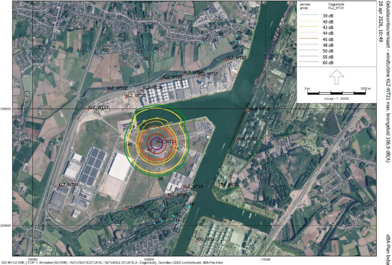
Figuur 3: Geluidscontourenkaart het project - max. brongeluid 106,9 dB(A) – luchtfoto ISO9613:2-2024
