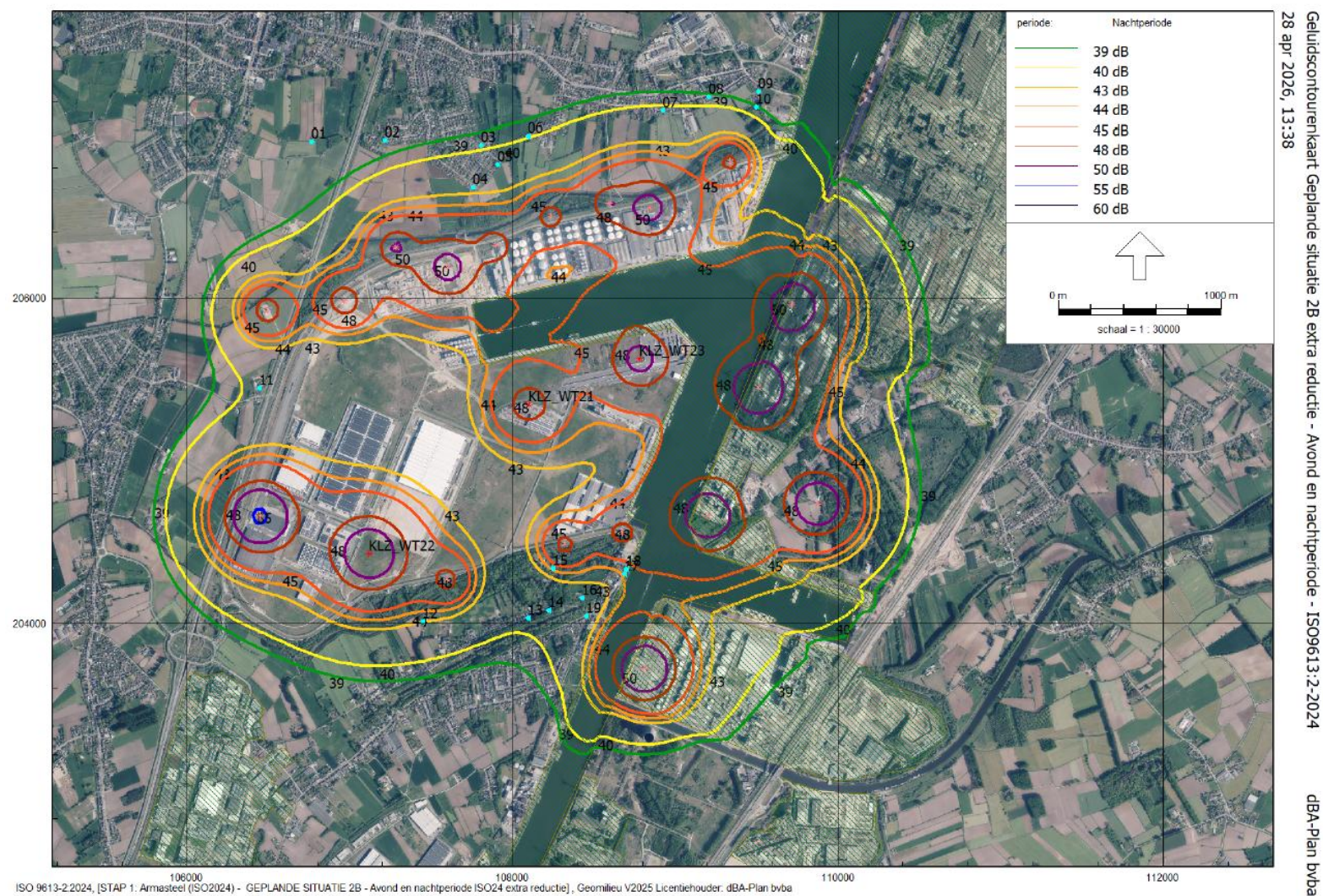
Figuur 18: Geluidscontourenkaart Geplande situatie 2B avond en nachtperiode extra reductie – luchtfoto ISO9613:2-2024
