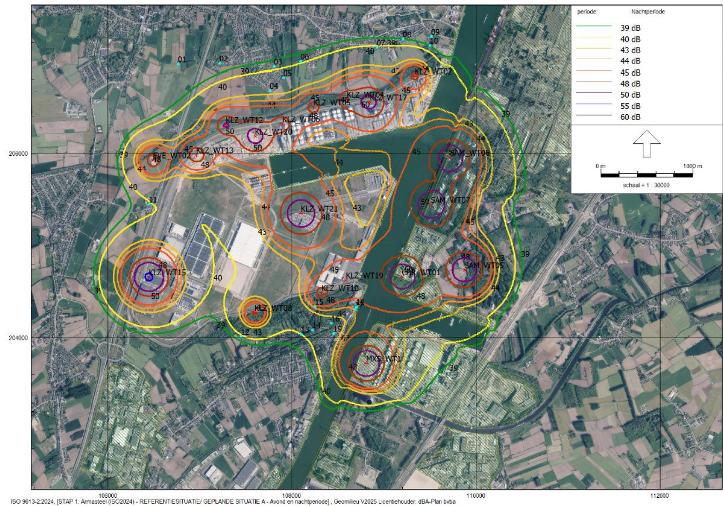
Figuur 9: Geluidscontourenkaart Geplande situatie 1A avond en nachtperiode – luchtfoto ISO9613:2-2024
