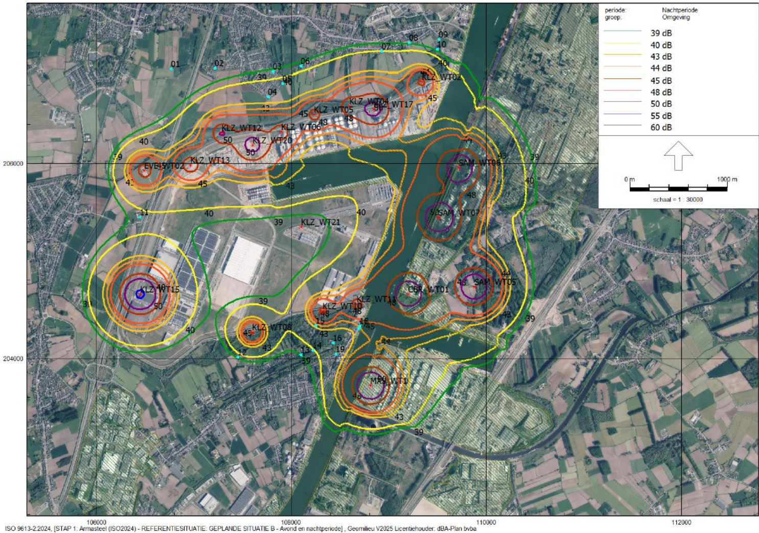
Figuur 7: Geluidscontourenkaart referentiesituatie B avond en nachtperiode – luchtfoto ISO9613:2-2024
