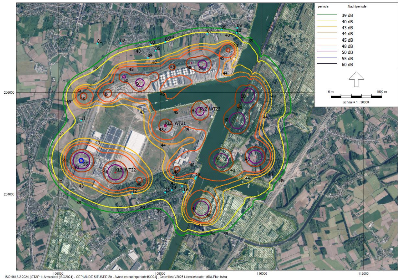
Figuur 15: Geluidscontourenkaart Geplande situatie 2A avond en nachtperiode – luchtfoto ISO9613:2-2024
