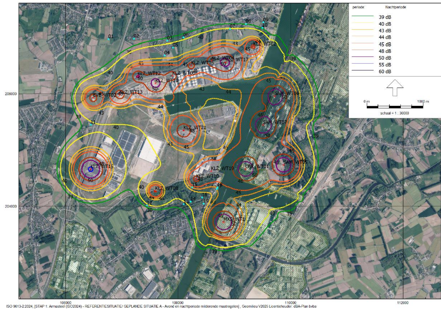
Figuur 10: Geluidscontourenkaart Geplande situatie 1A Milderende maatregelen - avond en nachtperiode – luchtfoto ISO9613:2-2024
