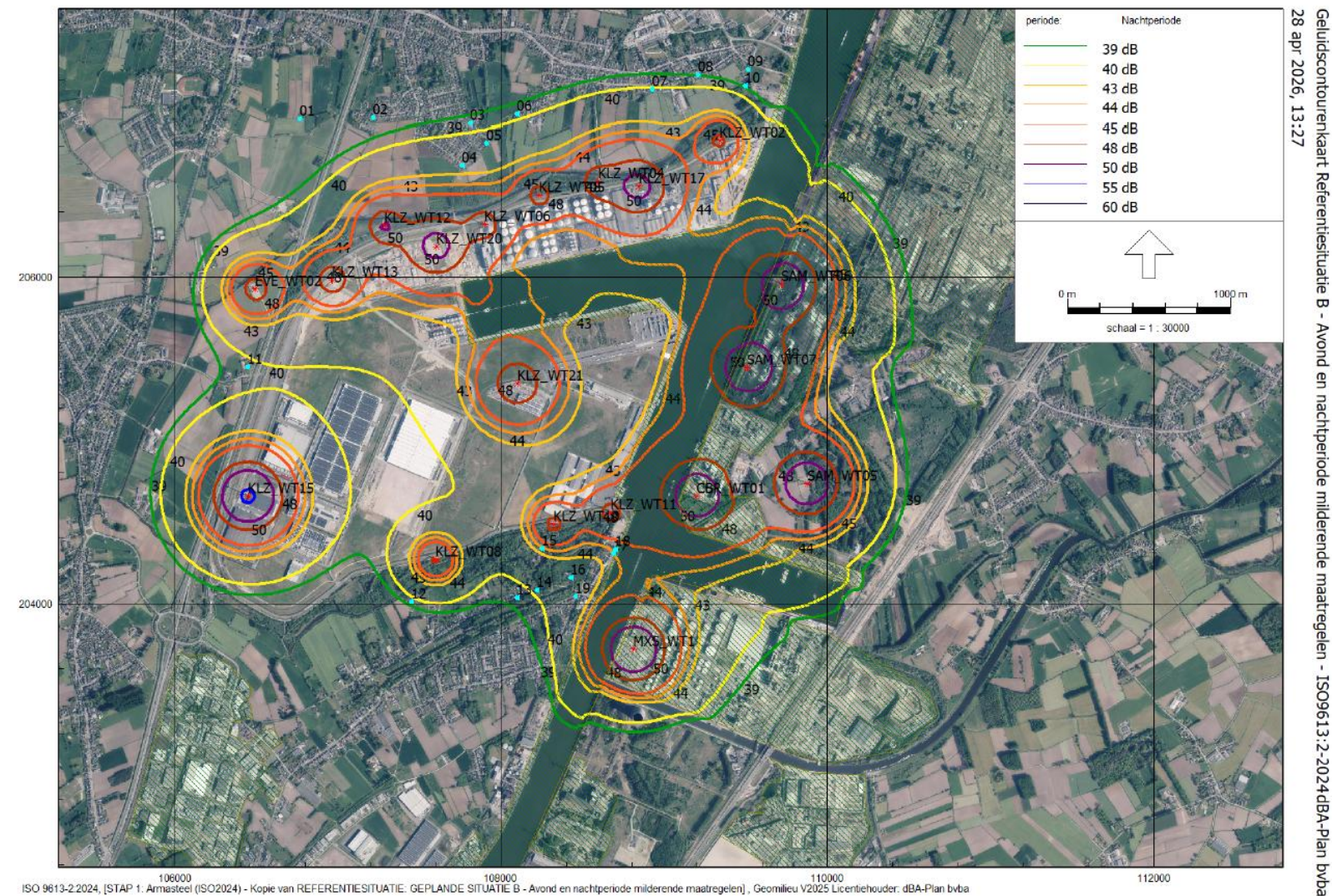
Figuur 13: Geluidscontourenkaart Geplande situatie 1B avond en nachtperiode na milderende maatregelen – luchtfoto ISO9613:2-2024
