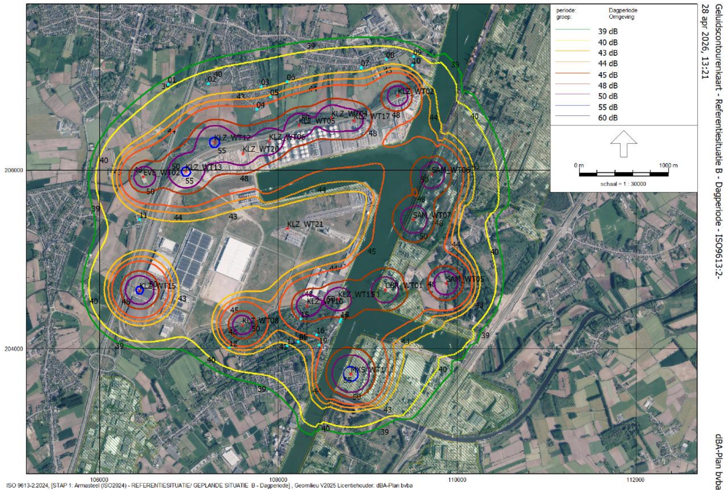
Figuur 6: Geluidscontourenkaart referentiesituatie B dagperiode – luchtfoto ISO9613:2-2024
