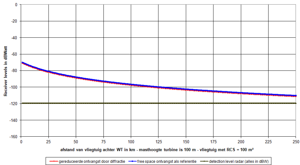
Reductie in zichtbaarheid door diffractie op WT - afstand radar tot WT is 26 km vlieghoogte = 1000 m (3000 ft)
