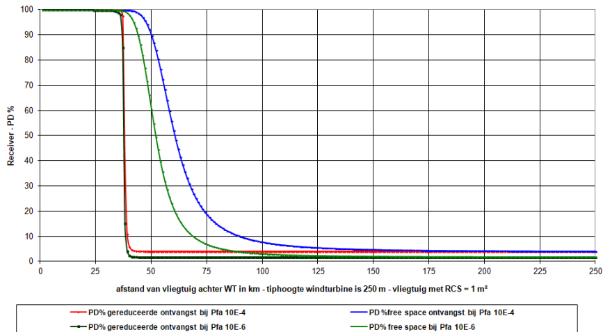
Reductie in zichtbaarheid door diffractie op WT - afstand radar tot WT is 25,4 km SW = 0 vlieghoogte = 600 m (2000 ft)
