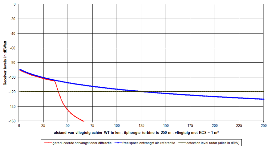
Reductie in zichtbaarheid door diffractie op WT - afstand radar tot WT is 25,4 km vlieghoogte = 600 m (2000 ft)
