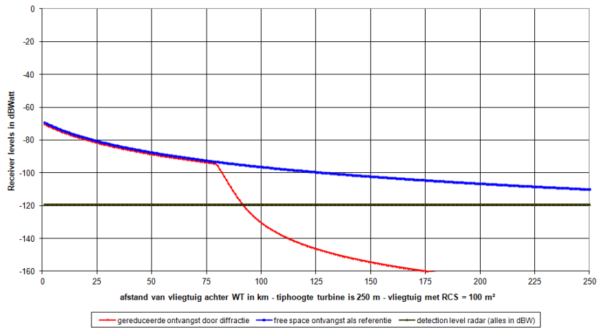
Reductie in zichtbaarheid door diffractie op WT - afstand radar tot WT is 25,4 km vlieghoogte = 1000 m (3000 ft)
