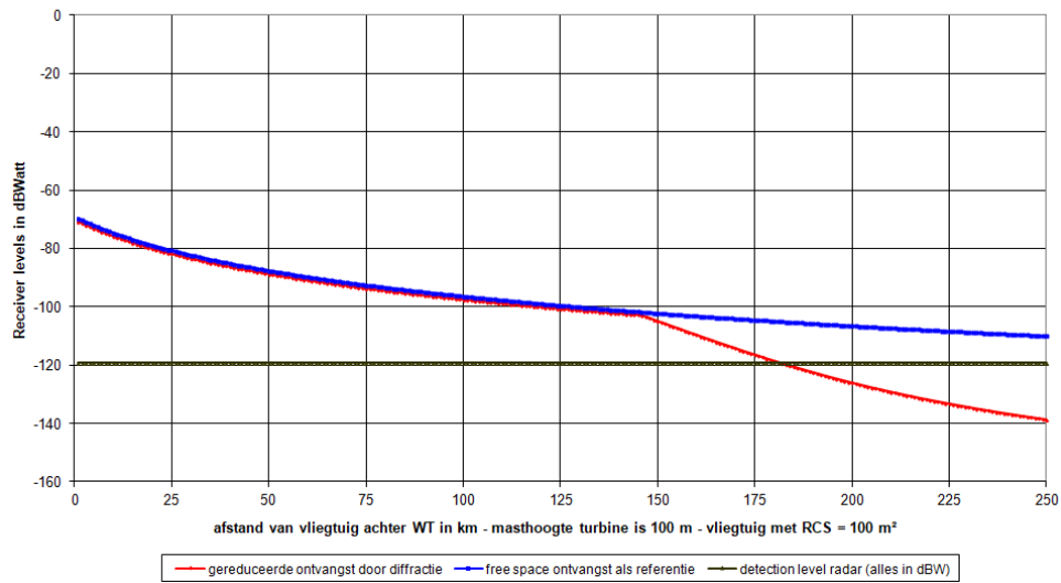
Reductie in zichtbaarheid door diffractie op WT - afstand radar tot WT is 26 km vlieghoogte = 600 m (2000 ft)
