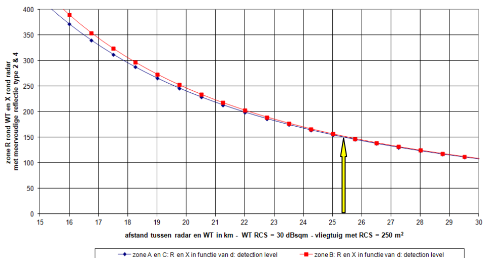
Type 2 en 4: zones rond windturbine R en radar X in functie van afstand d bij een detectielevel van -119 dBW
