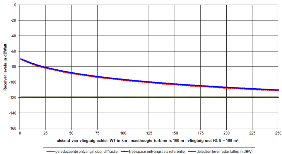
Reductie in zichtbaarheid door diffractie op WT - afstand radar tot WT is 26 km vlieghoogte = 3000 m (10000 ft)
