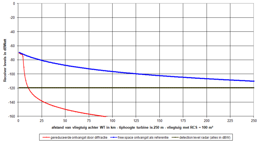
Reductie in zichtbaarheid door diffractie op WT - afstand radar tot WT is 25,4 km vlieghoogte = 300 m (1000 ft)
