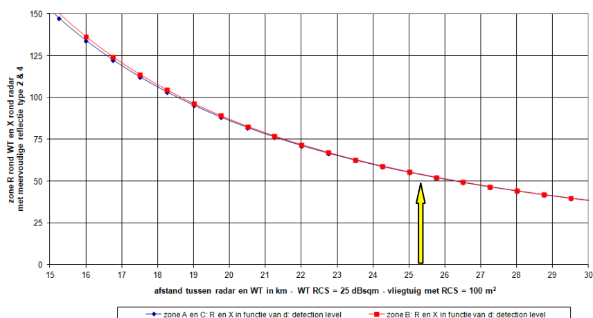
Type 2 en 4: zones rond windturbine R en radar X in functie van afstand d bij een detectielevel van -119 dBW
