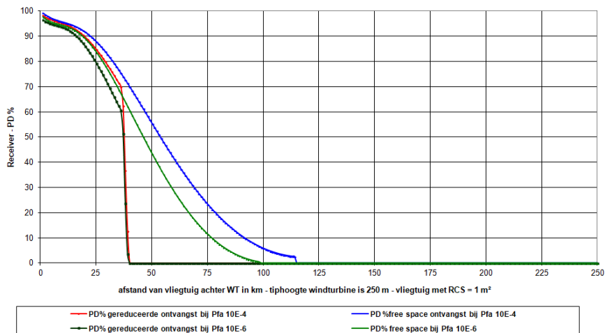
Reductie in zichtbaarheid door diffractie op WT - afstand radar tot WT is 25,4 km SW = 1 vlieghoogte = 600 m (2000 ft)
