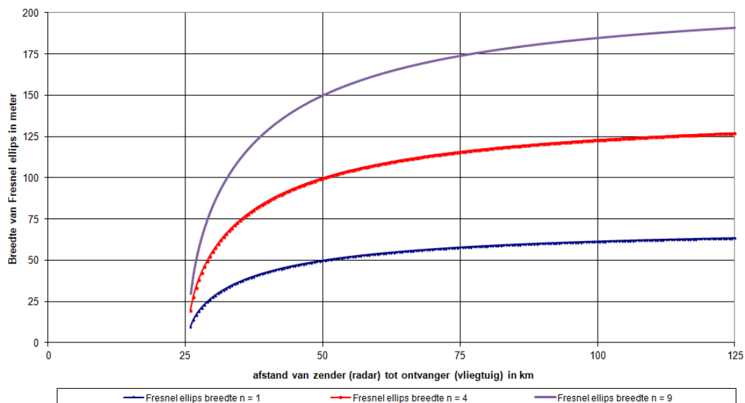
Fresnel ellips breedte ter hoogte van de windturbines afstand van zendantenne tot windturbine = 25,4 km
