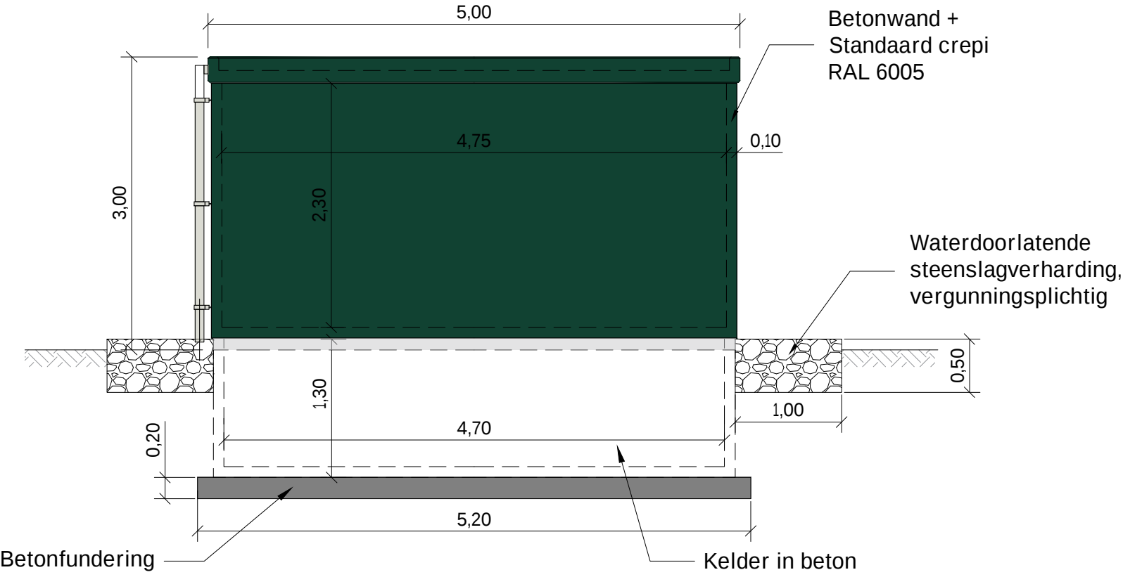
ACHTERAANZICHT
