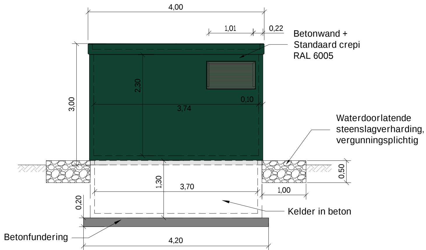
LINKERAANZICHT
