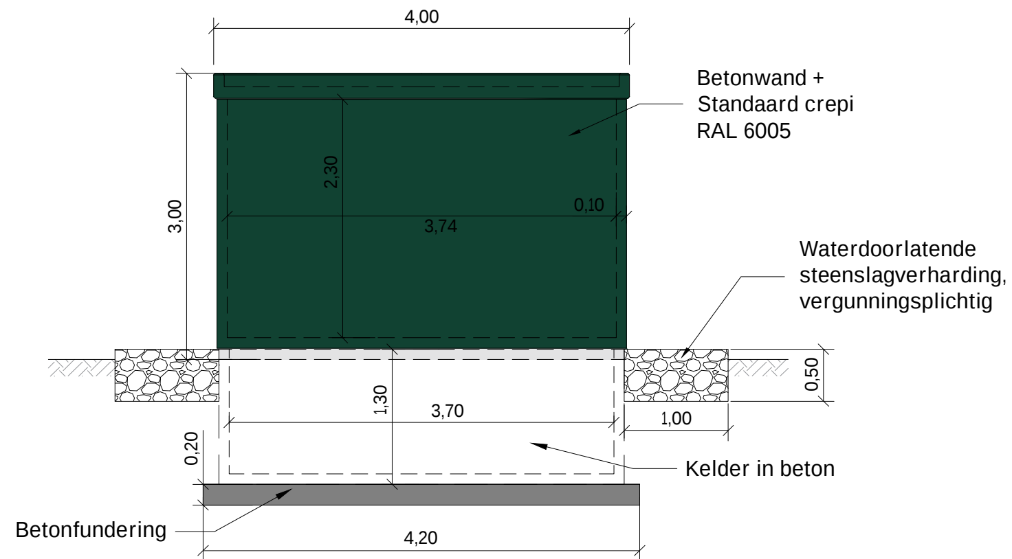
RECHTERAANZICHT
