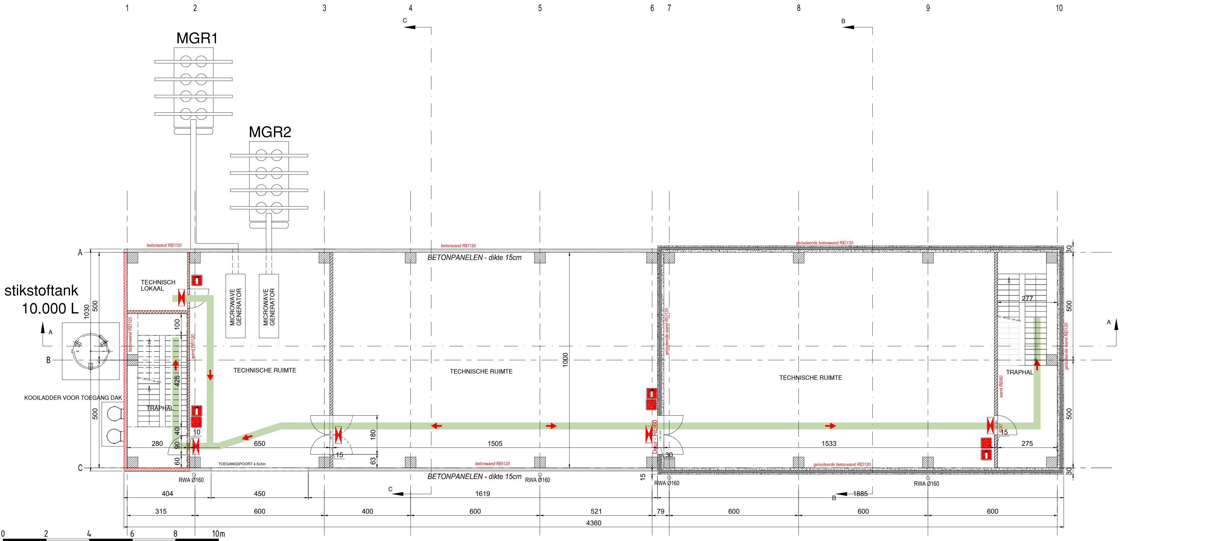
0 2 4 6 8 10m schaal: 1/100 BA_OPERATIONEEL GEBOUW_PB_N_02_NIVEAU +01
