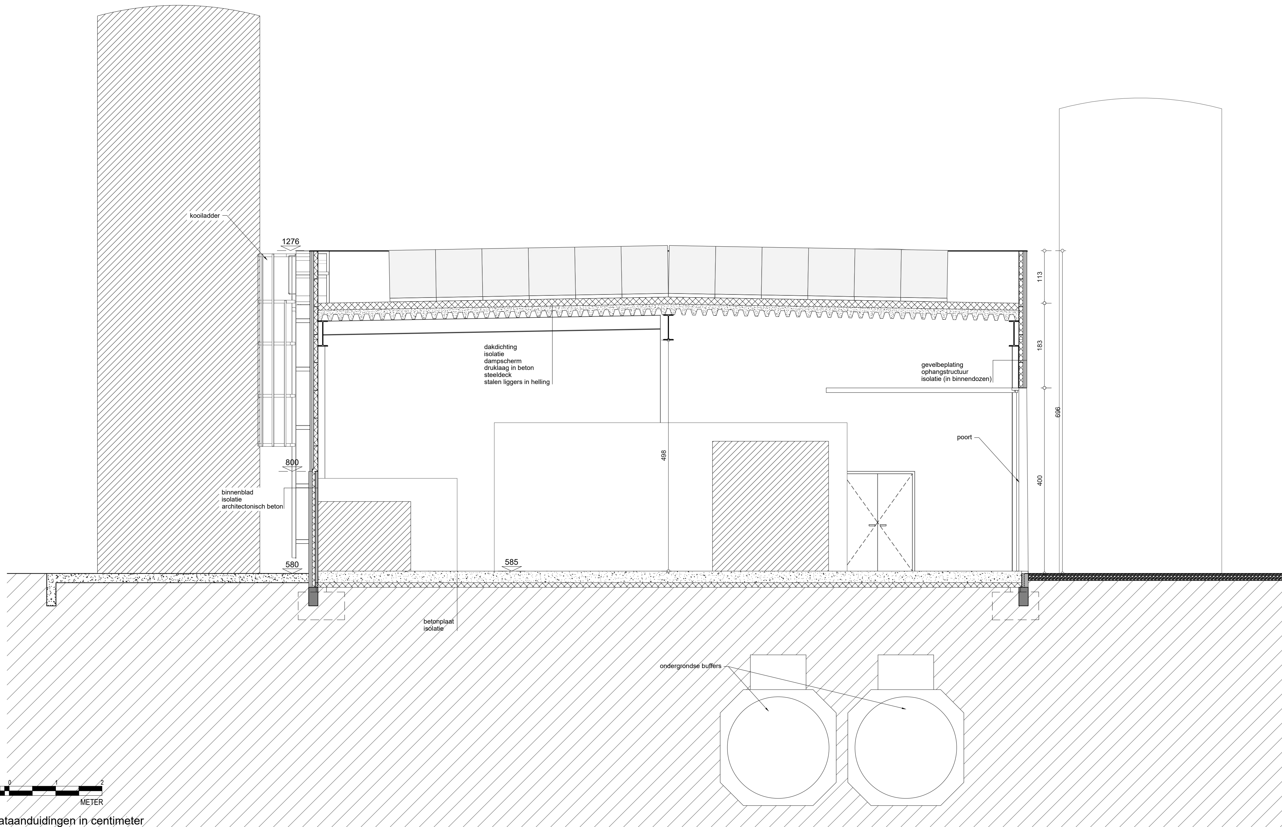
Maataanduidingen in centimeter Referentiepeil in T.A.W. BA_GEBOUW_SB_N_01_snedes A
