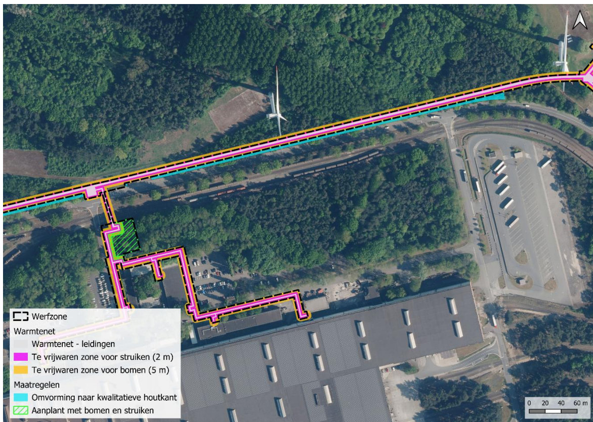
Figuur 3-3: Aanduiding van te vrijwaren zones om schade aan de leidingen te voorkomen door bomen/struiken en aanduiding van de zones waar heraanplant van bomen en struiken mogelijk is – in het oosten van het projectgebied
