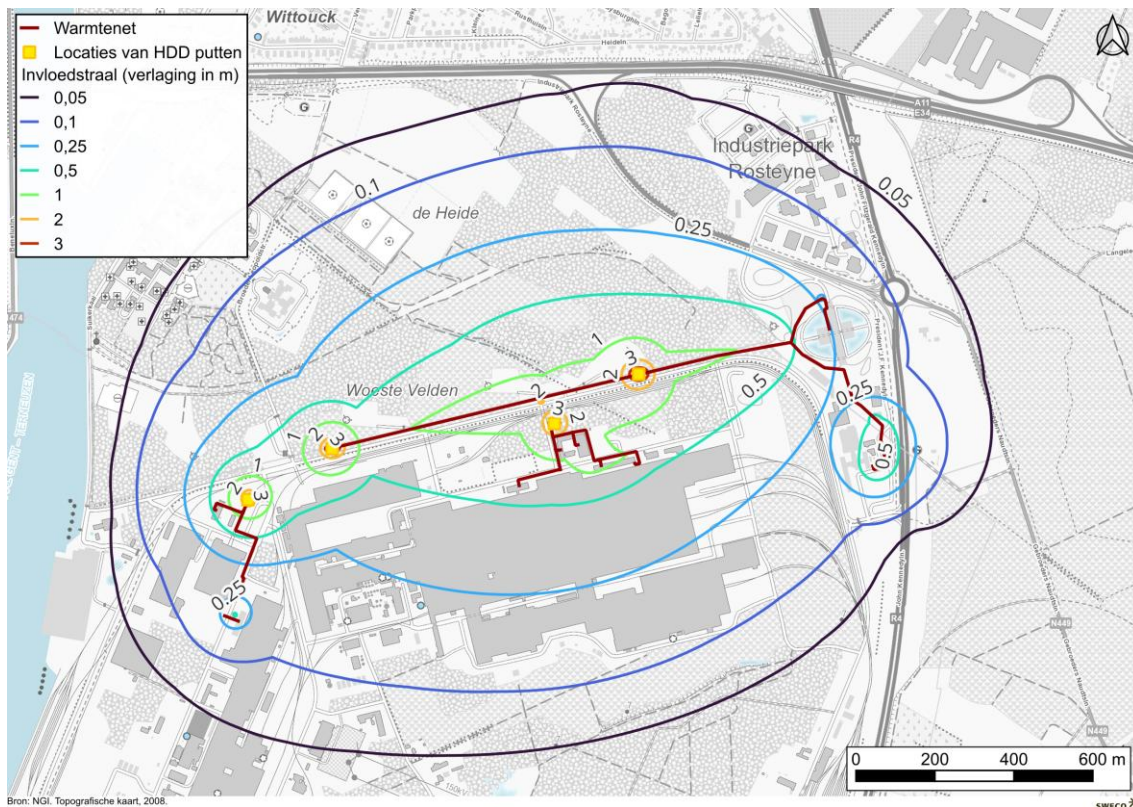
Figuur 1-3: Maximale verlagingscontour tgv de grondwaterbemaling
