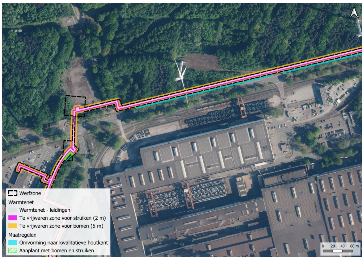
Figuur 3-1: Aanduiding van te vrijwaren zones om schade aan de leidingen te voorkomen door bomen/struiken en aanduiding van de zones waar heraanplant van bomen en struiken mogelijk is – in het westen van het projectgebied
