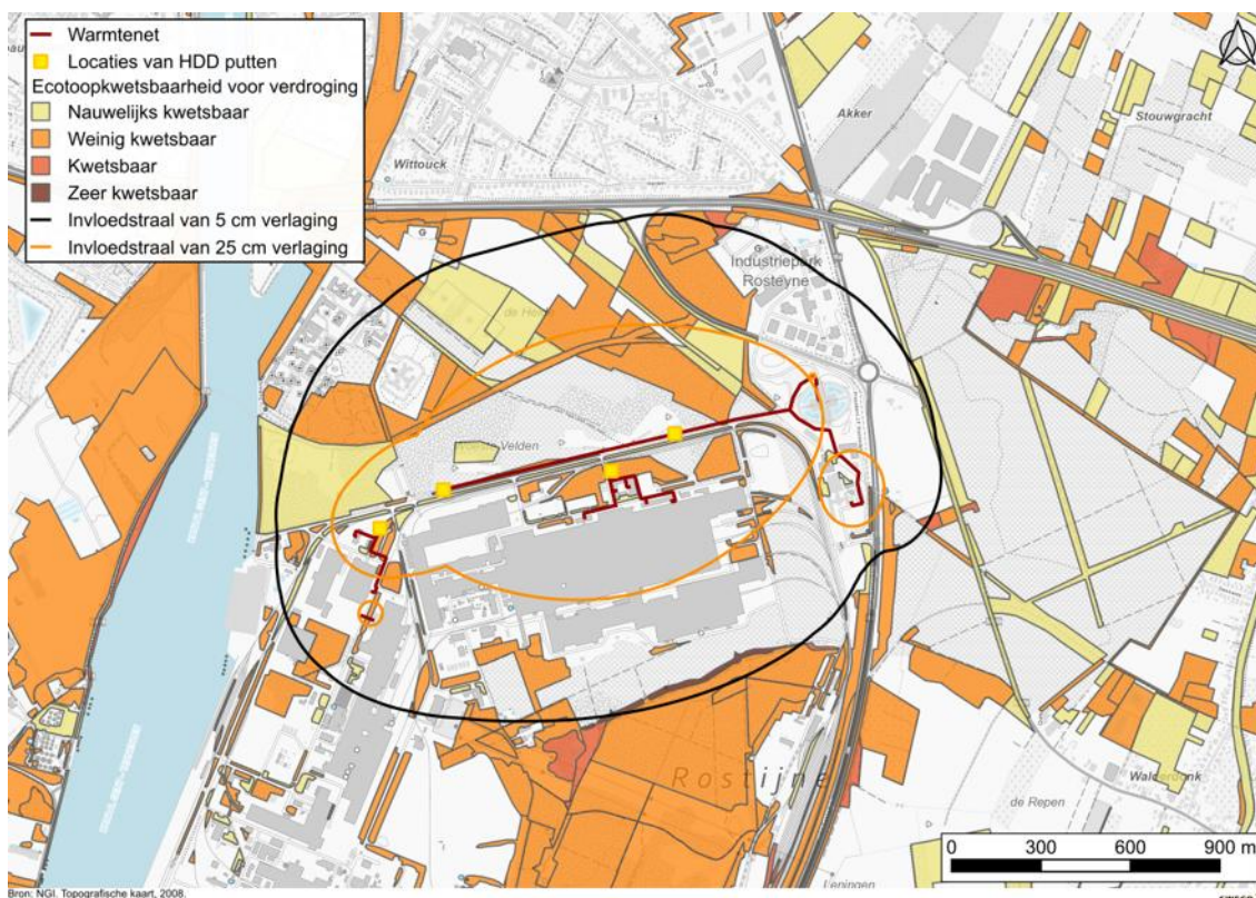
Figuur 3-4: Invloedstraal t.o.v. de ecotoopkwetsbaarheid voor droogte, versie 2025.
