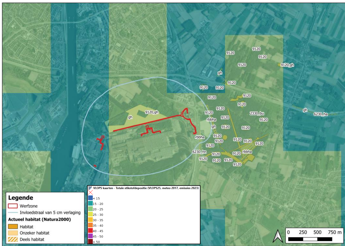
Figuur 2-9: Totale stikstofdepositie volgens VLOPS25 ter hoogte van het projectgebied
