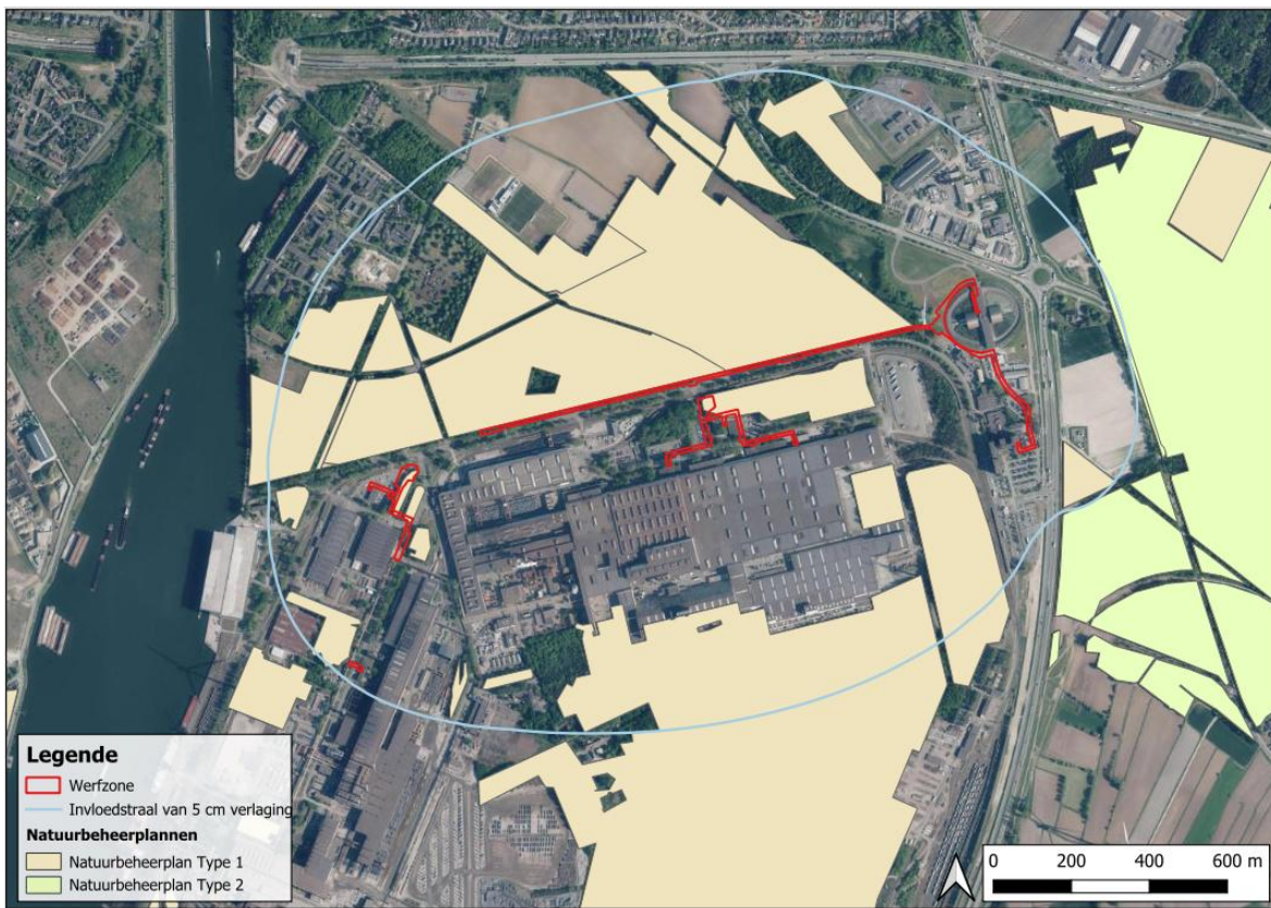
Figuur 2-2: Situering Natuurbeheerplan type thv de werfzone
