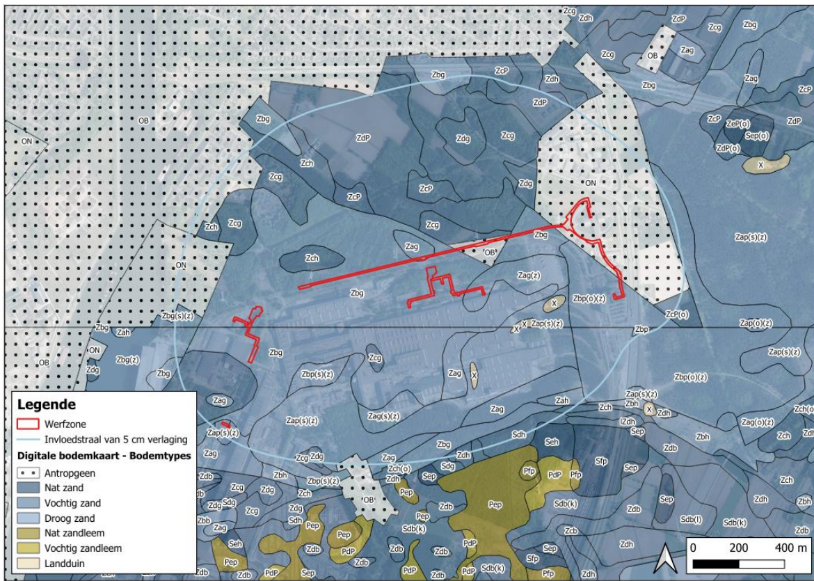
Figuur 2-8: Bodemtypes ter hoogte van het projectgebied met aanduiding van de bemalingscontour.
