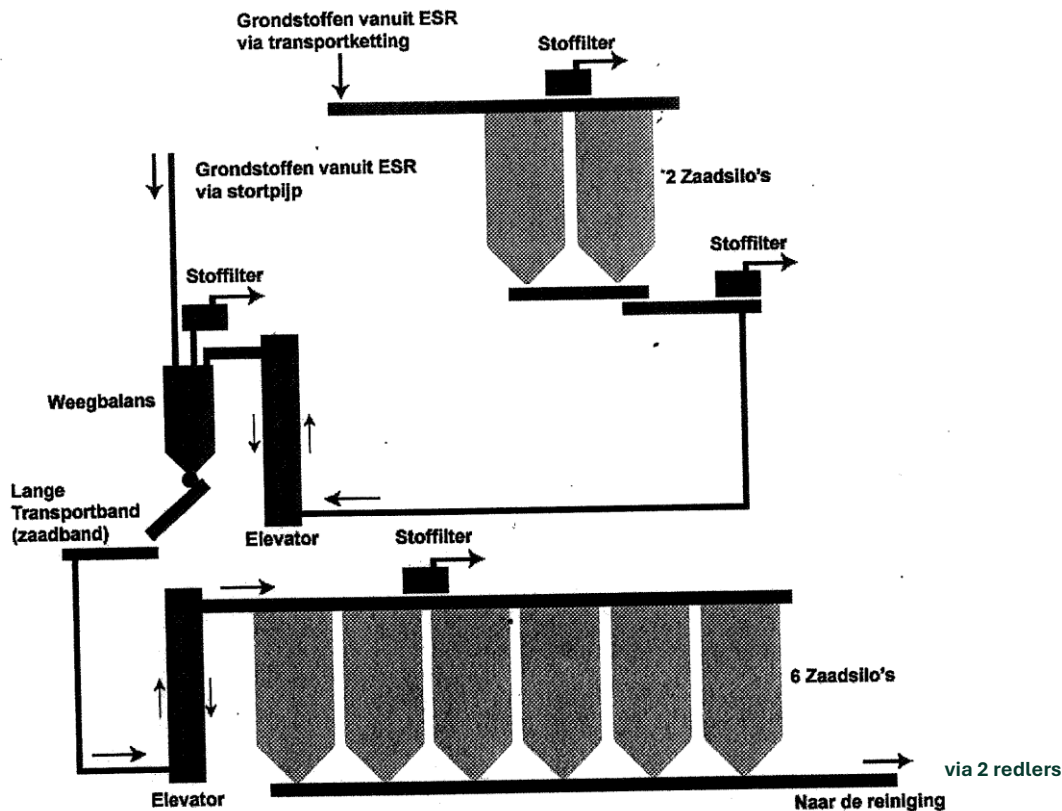
Figuur 2: Transportsystemen van de grondstoffen met aanduiding van maatregelen ter beperking van diffuse stofemissies
