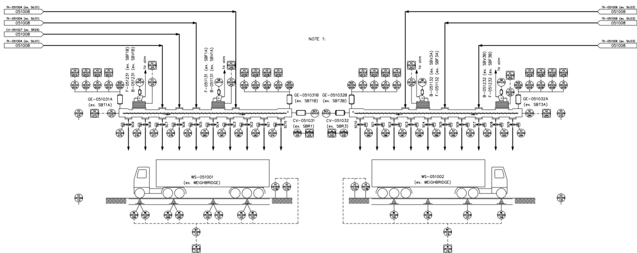
Figuur 8: processchema vrachtwagenbelading
