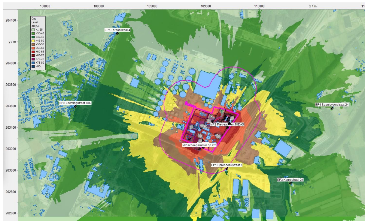
Figuur XIII-11: Geluidscontourkaart van de geluidsbelasting van de totale inrichting, toekomstige situatie
