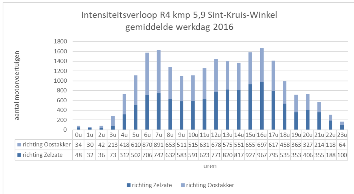
Figuur XV-4: Intensiteitsverloop R4 ten noorden van het kruispunt met de Moervaartkaai, mvt per uur (bron: AWW).
