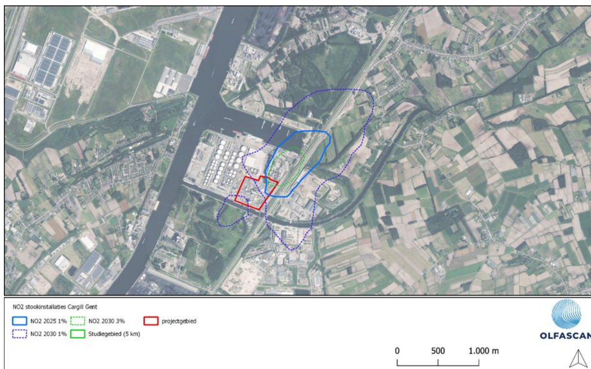
Figuur X-6: Impact NO 2 Cargill - toetsing aan huidige en toekomstige emissiegrenswaarden
