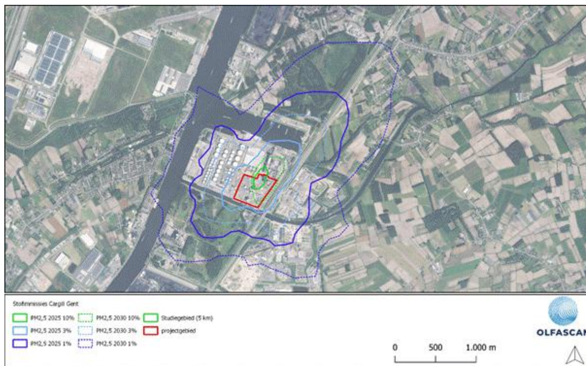
Figuur X-7: Impact PM 2,5 Cargill - modellerings emissies 'calamiteit'
