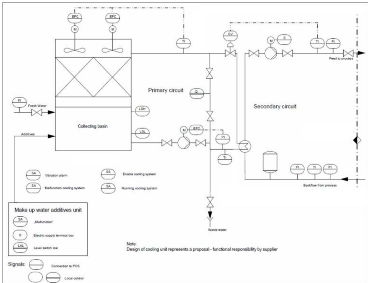
Figuur IV-11: stroomschema koeltoren
