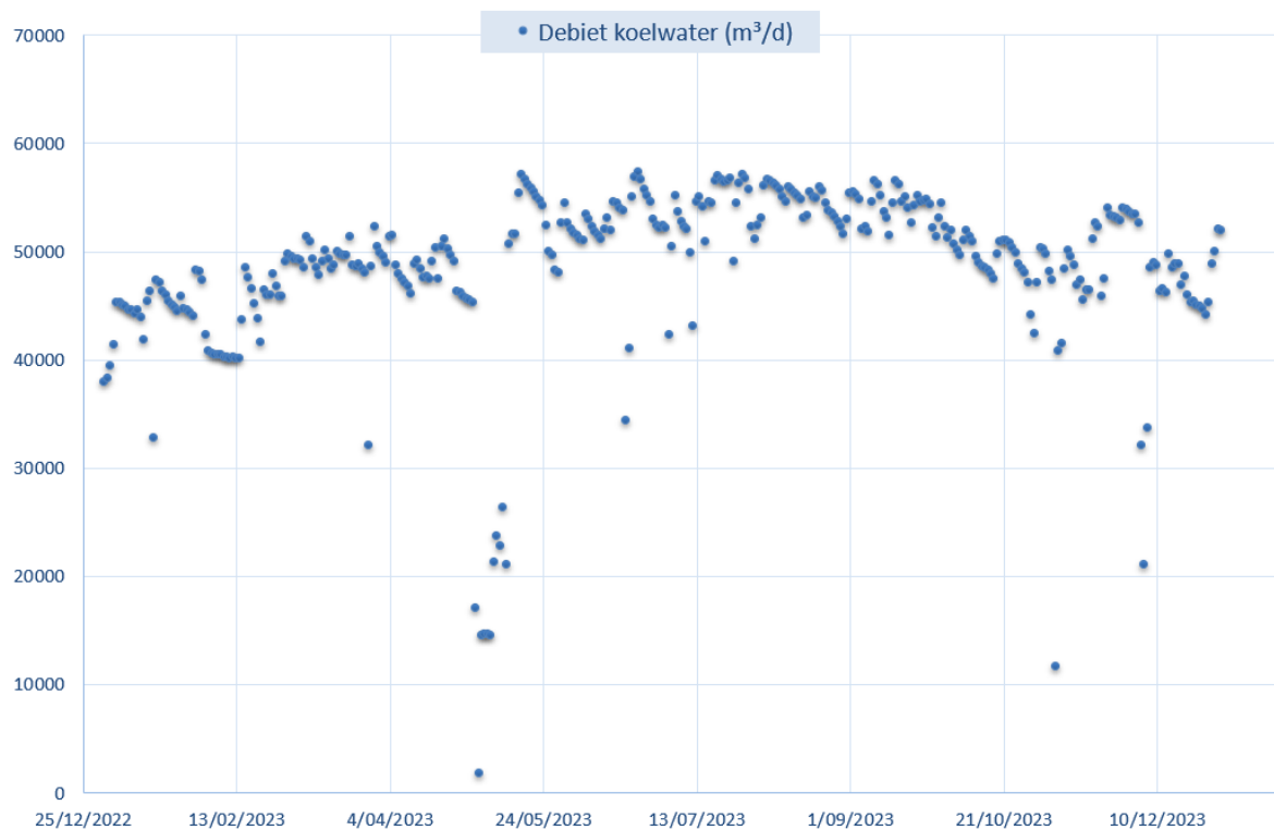
Figuur XI-8: Verloop koelwaterdebiet in 2023 (in m³/d)
