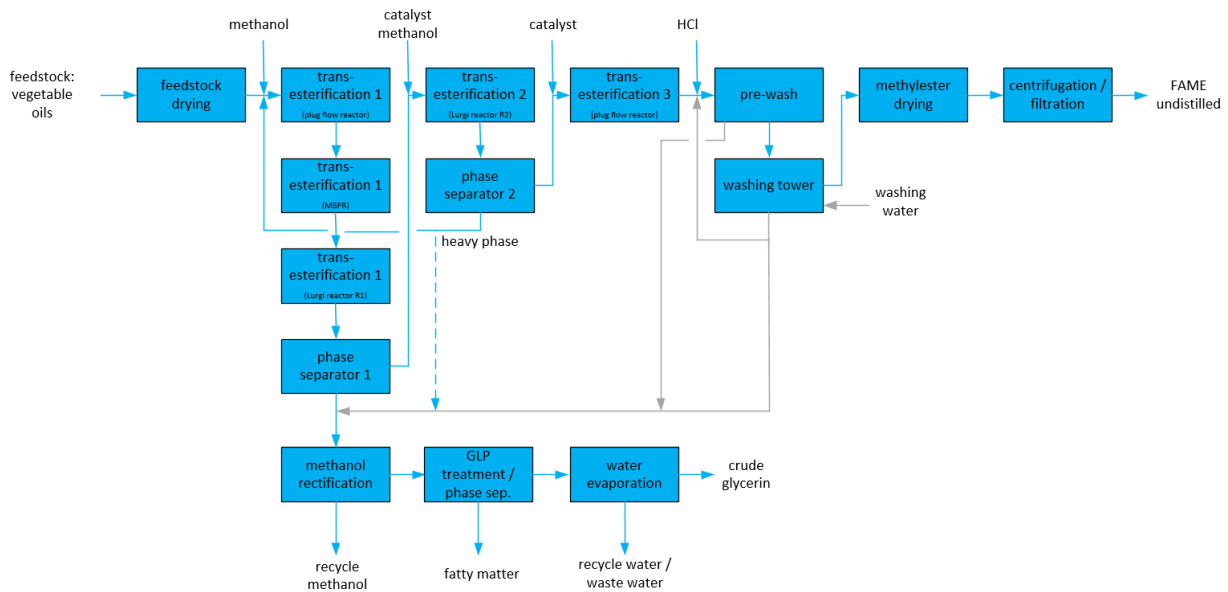
Figuur IV-4: Schematische voorstelling van de (1ste generatie) biodieselininstallatie
