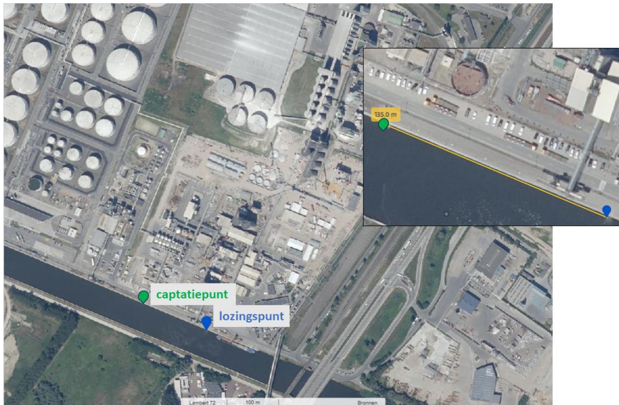
Figuur XI-7: Ligging captatie- en lozingspunt koelwater op Moervaart
