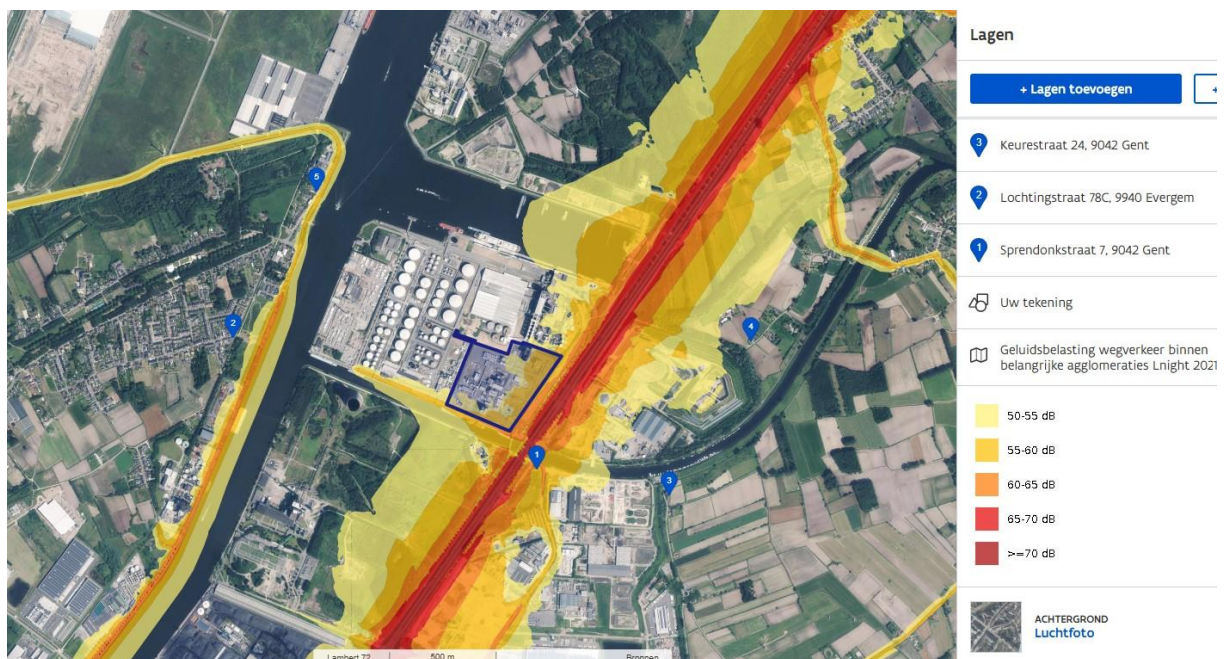
Figuur XIII-5: Strategische geluidsbelastingskaart Lnight wegverkeer, dd. 2021 (bron Geopunt Vlaanderen).
