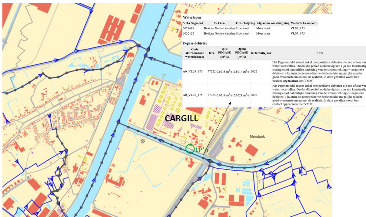
Figuur XI-4: Gegegreerd debiet via Pegasemodellering (Geoloket VMM).
