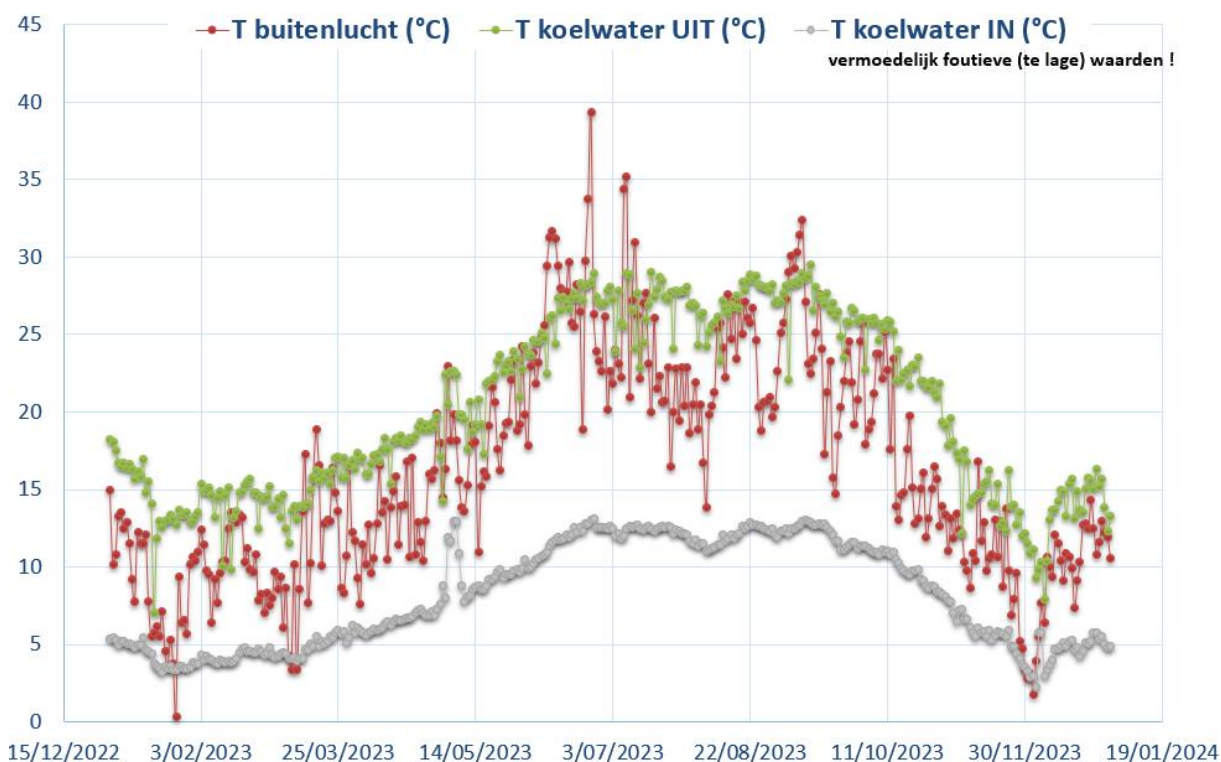
Figuur XI-9: Verloop temperatuur koelwaterinname, lozing koelwater en buitentemperatuur in 2023 (alles in °C) o.b.v. metingen Cargill – Bemerk dat de waarden voor koelwaterinname vermoedelijk foutieve metingen betreffen – zie aangepaste Figuur XI-10.
