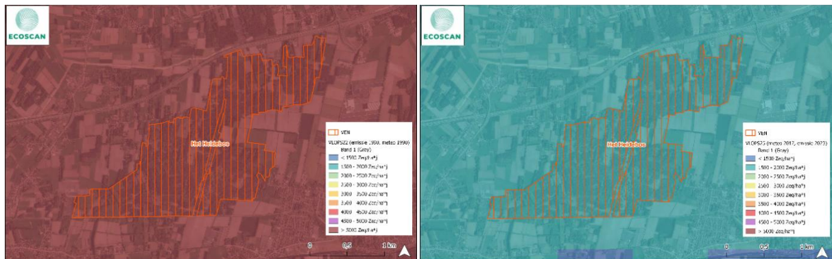
Figuur XIV-18: Evolutie van de verzurende depositie ter hoogte van het dichtstbijgelegen onderdeel van het VEN-gebied “Het Heidebos” o.b.v. VLOPS22 (emissie 1990, meteo 1990) (links), VLOPS25 (emissie 2023, meteo 2017) (rechts)
