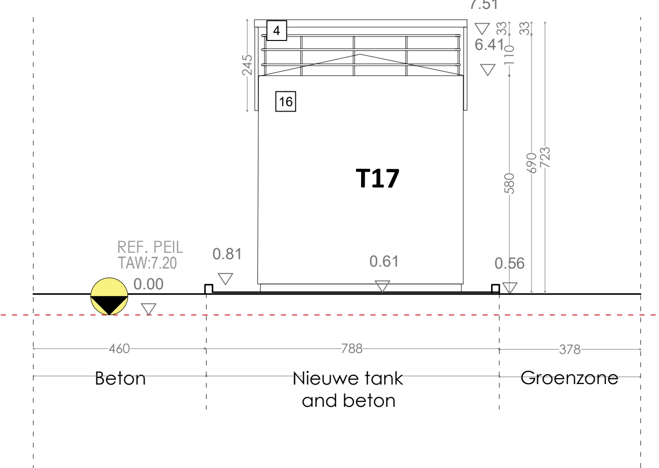
Gevel Rechts- G32
