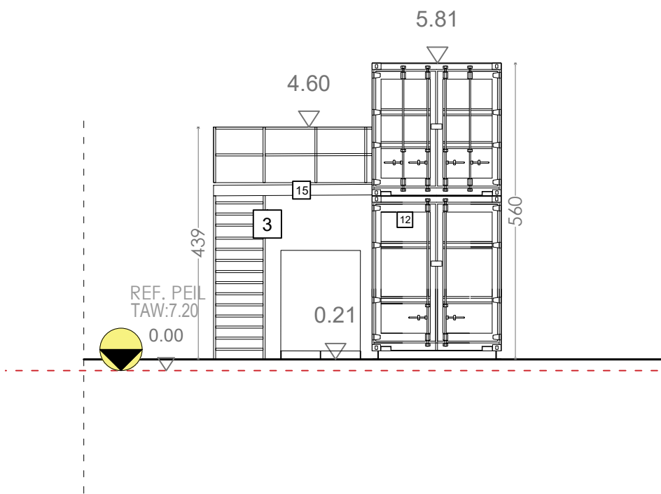
Achtergevel-G28
