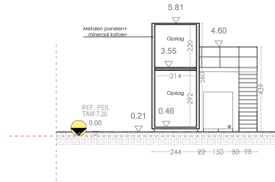
Snede - EE
