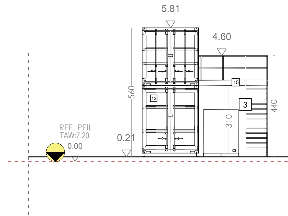
Voorgevel- G26
