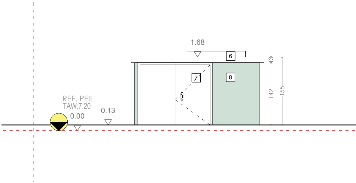
Vorgevel- G17
