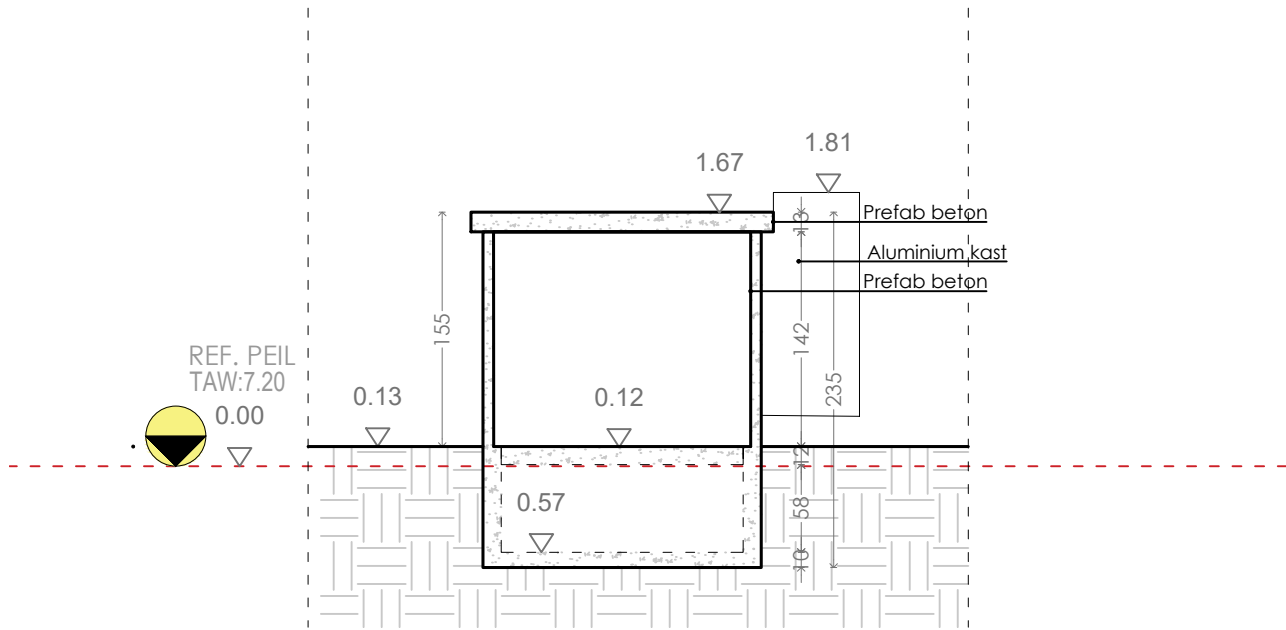
Sneede -GG
