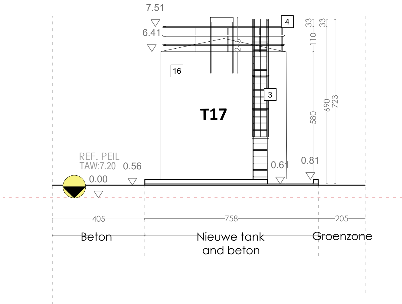
Voorgevel- G29
