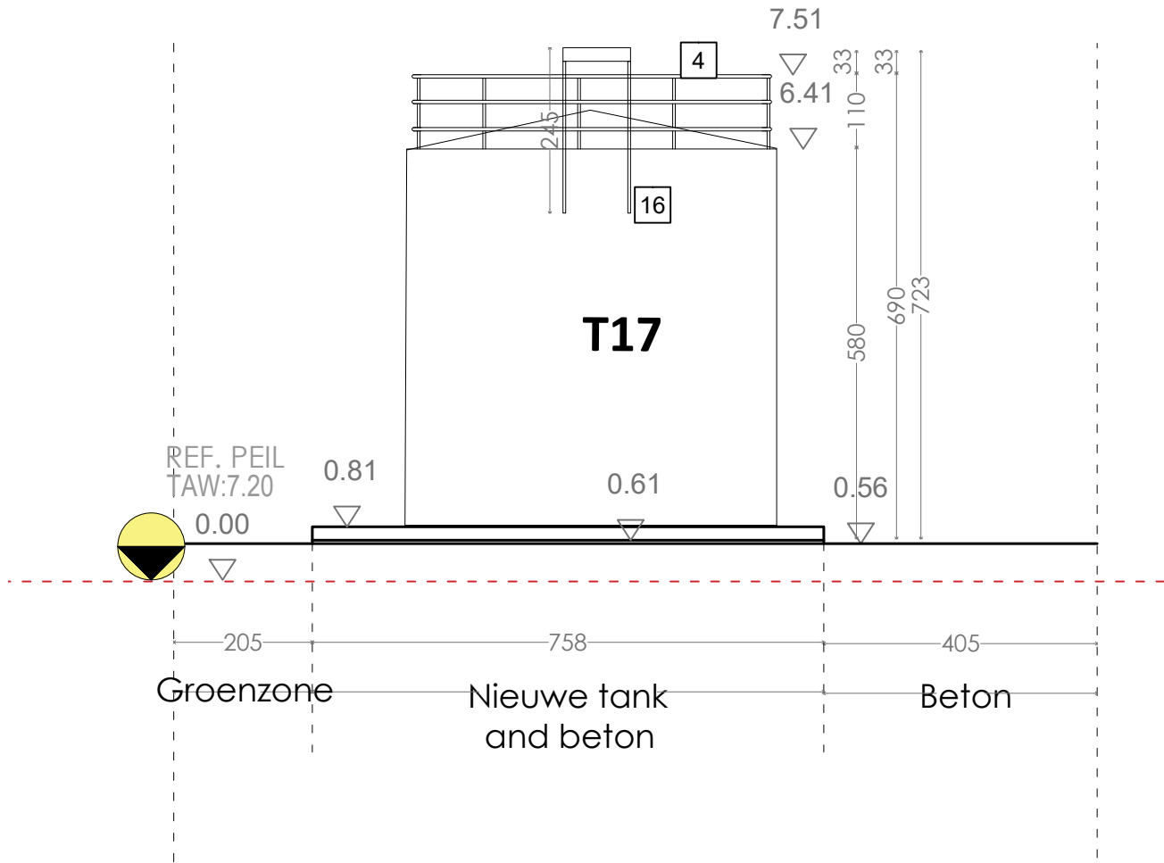
Achtergevel- G31
