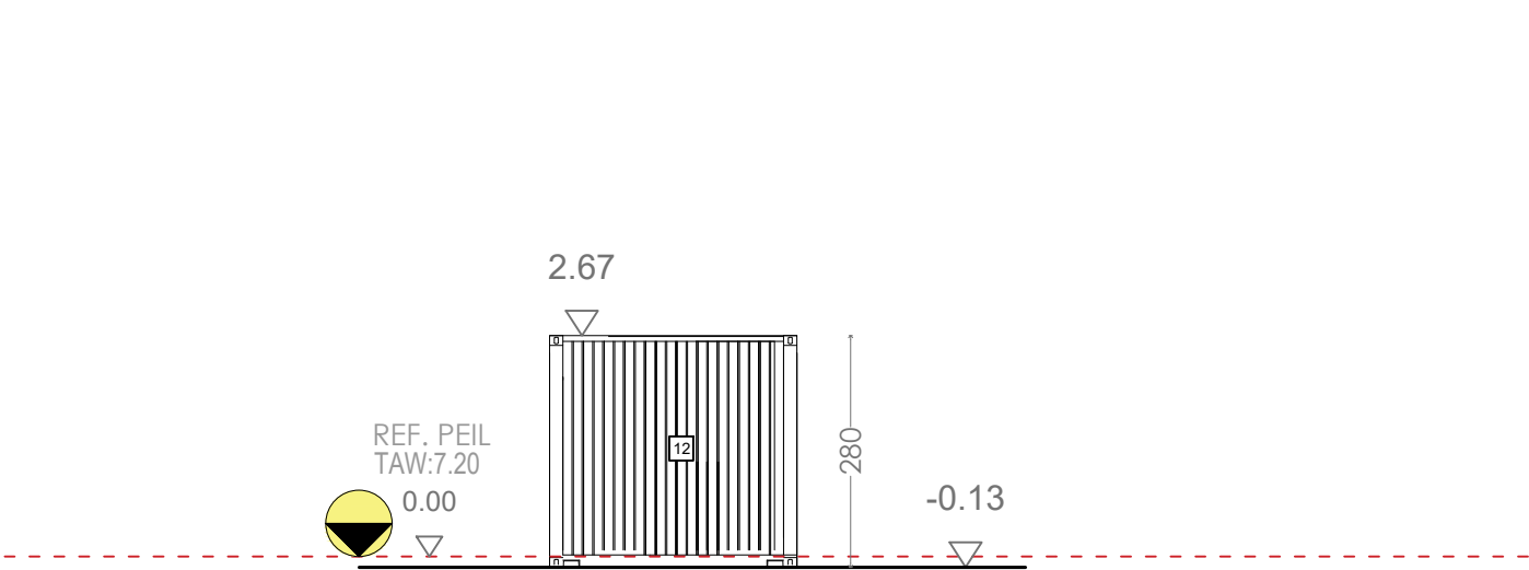
Achtergevel-G11
