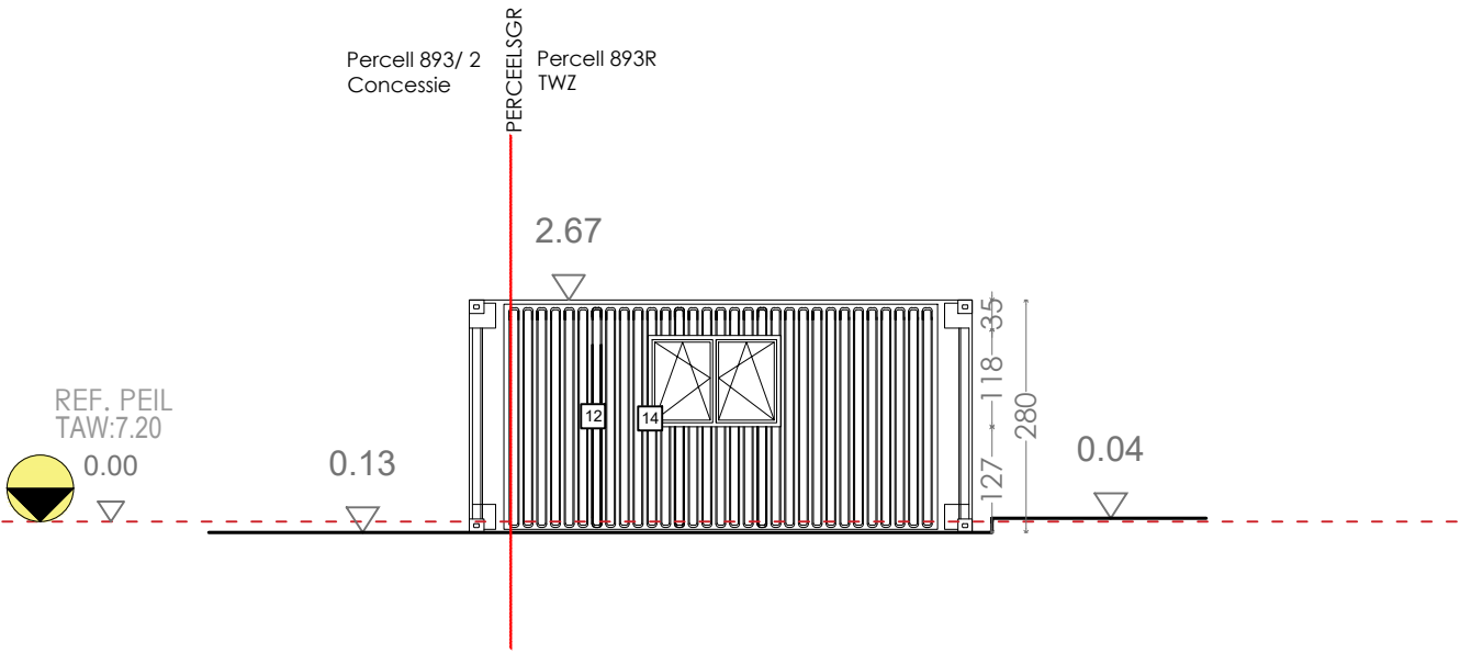
Zijgevel Rechts-G12
