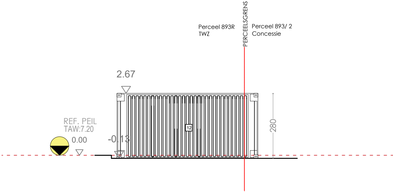
Zijgevel Links-G10
