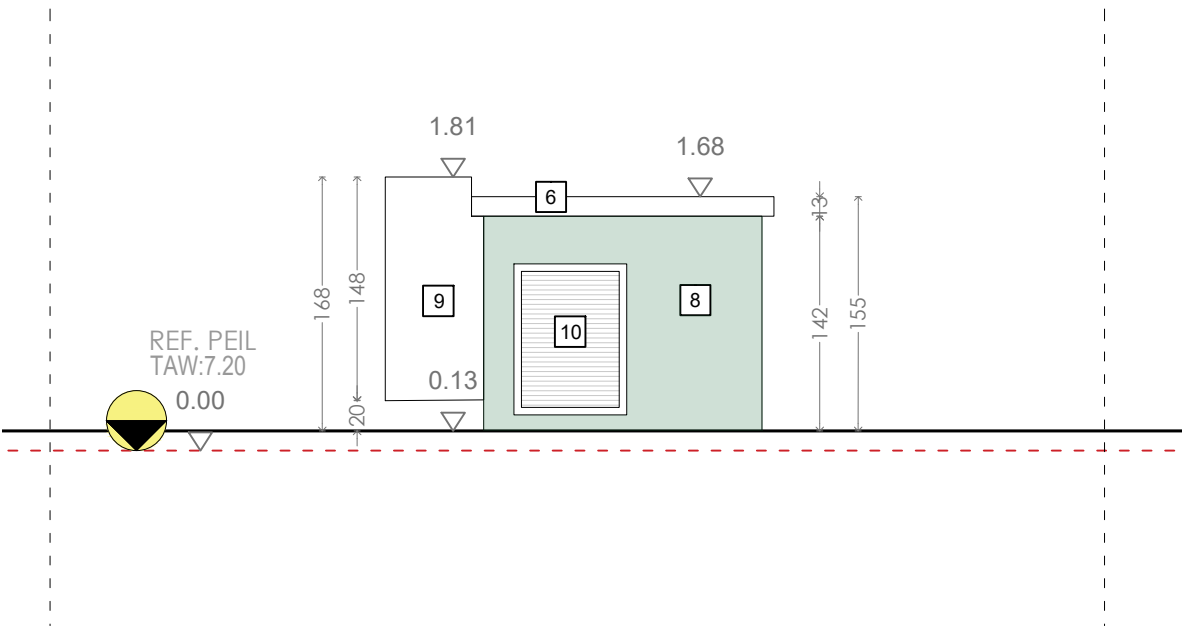
Gewel Links -G18
