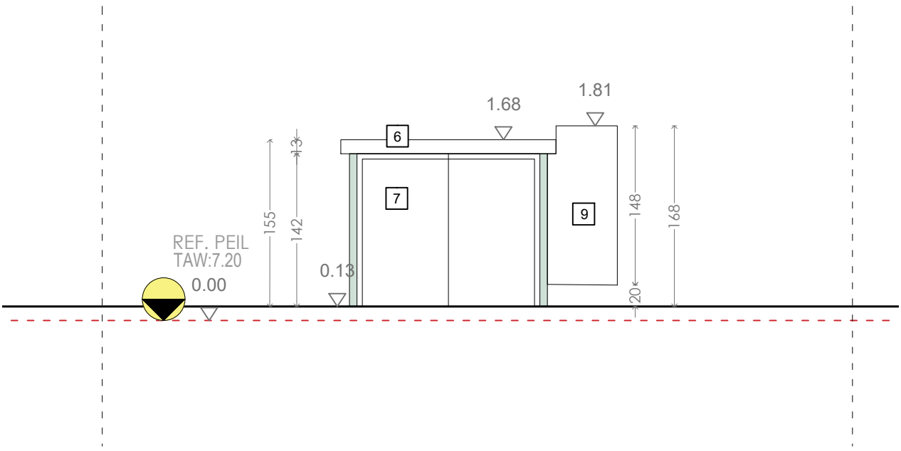
Gewel Rechts -G20
