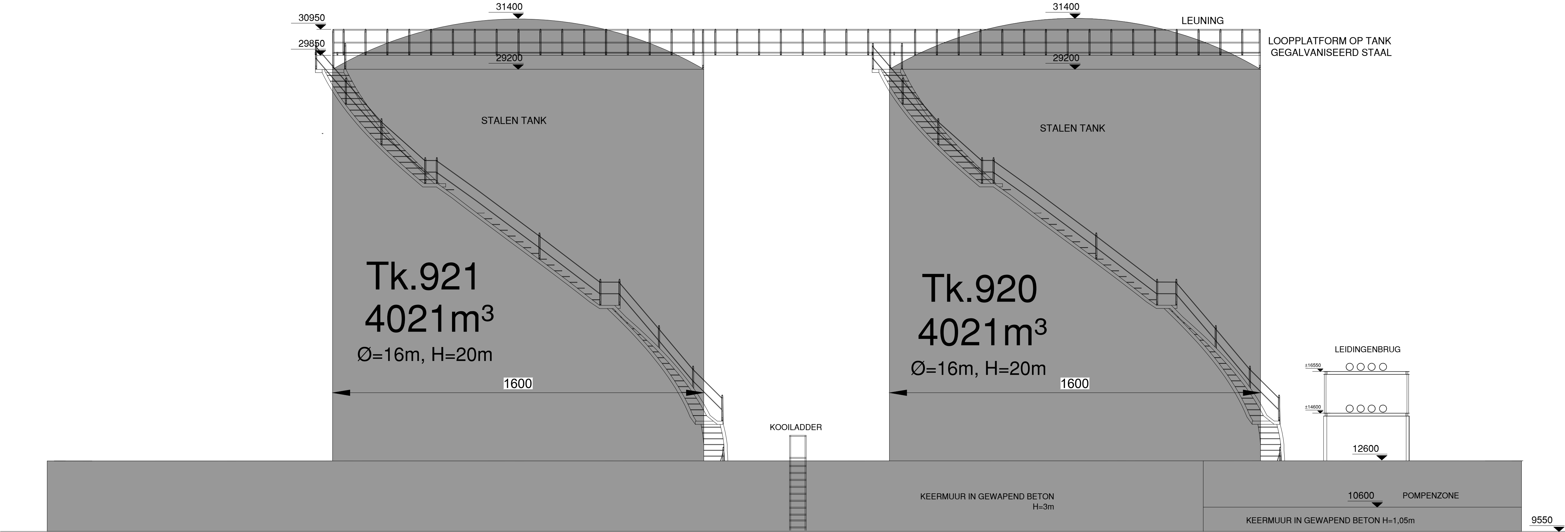
ZICHT OOSTEN TANKPARK L
