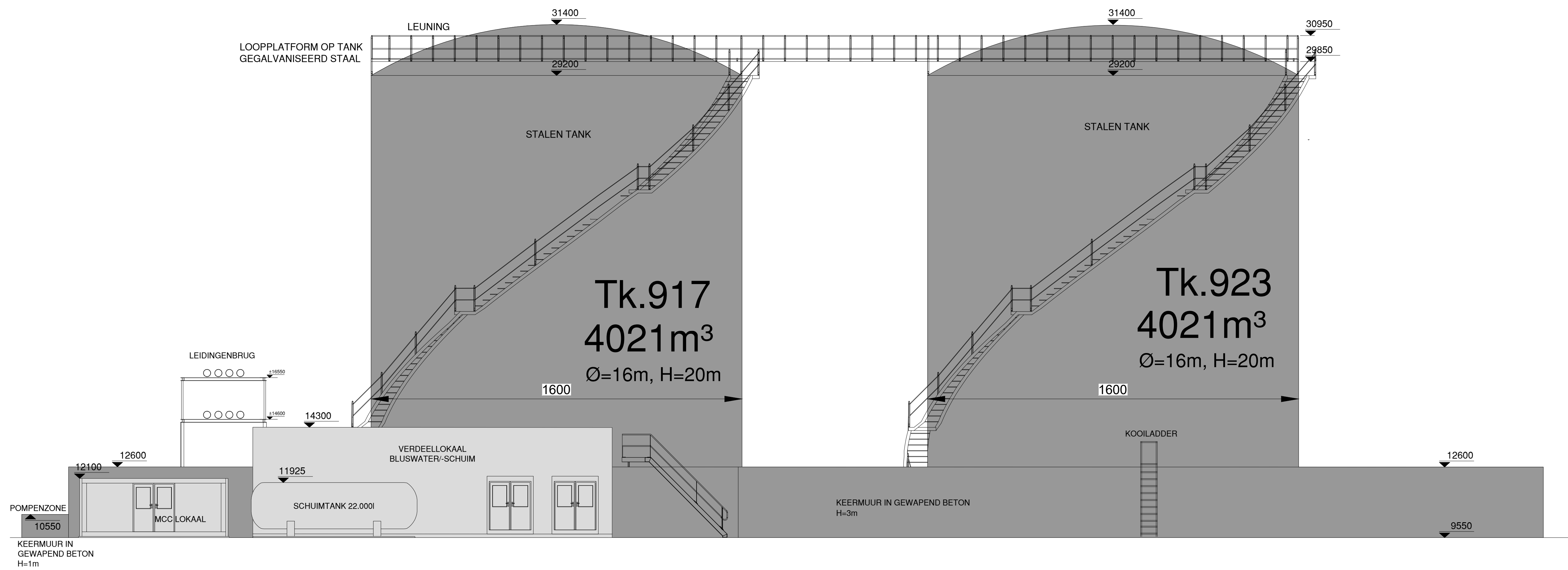
ZICHT WESTEN TANKPARK L
