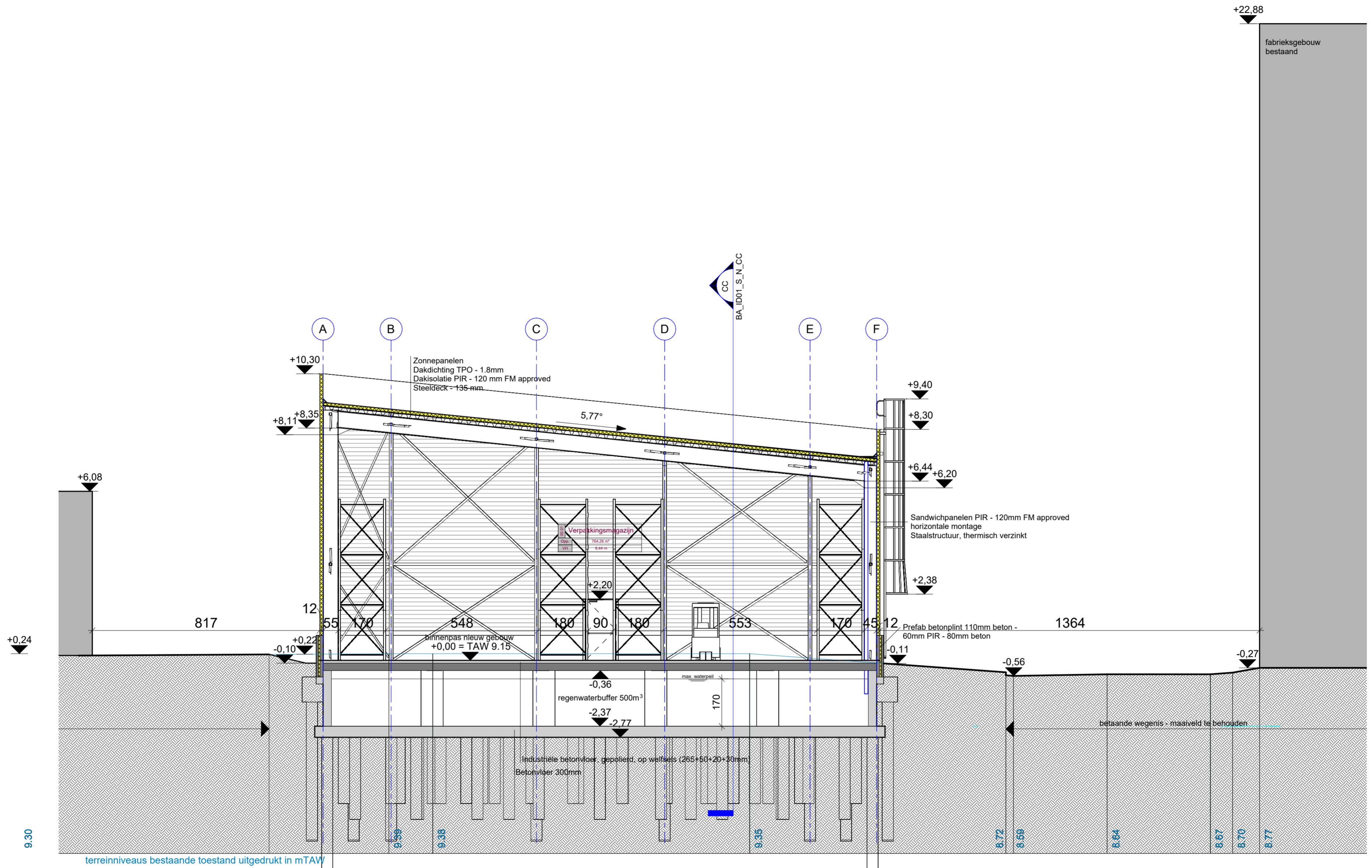
ID01 NT Doorsnede AA
