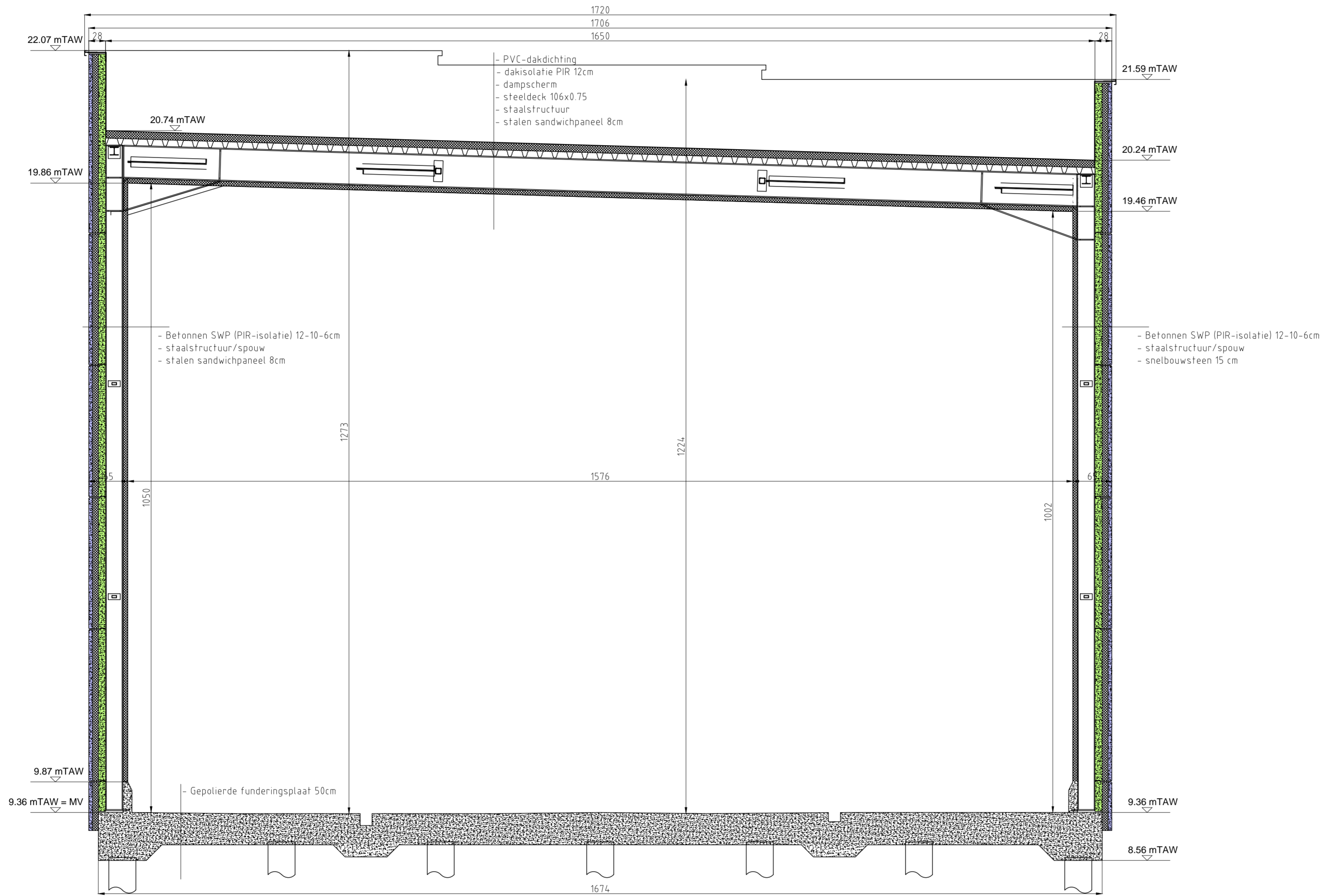
Snede B-B
