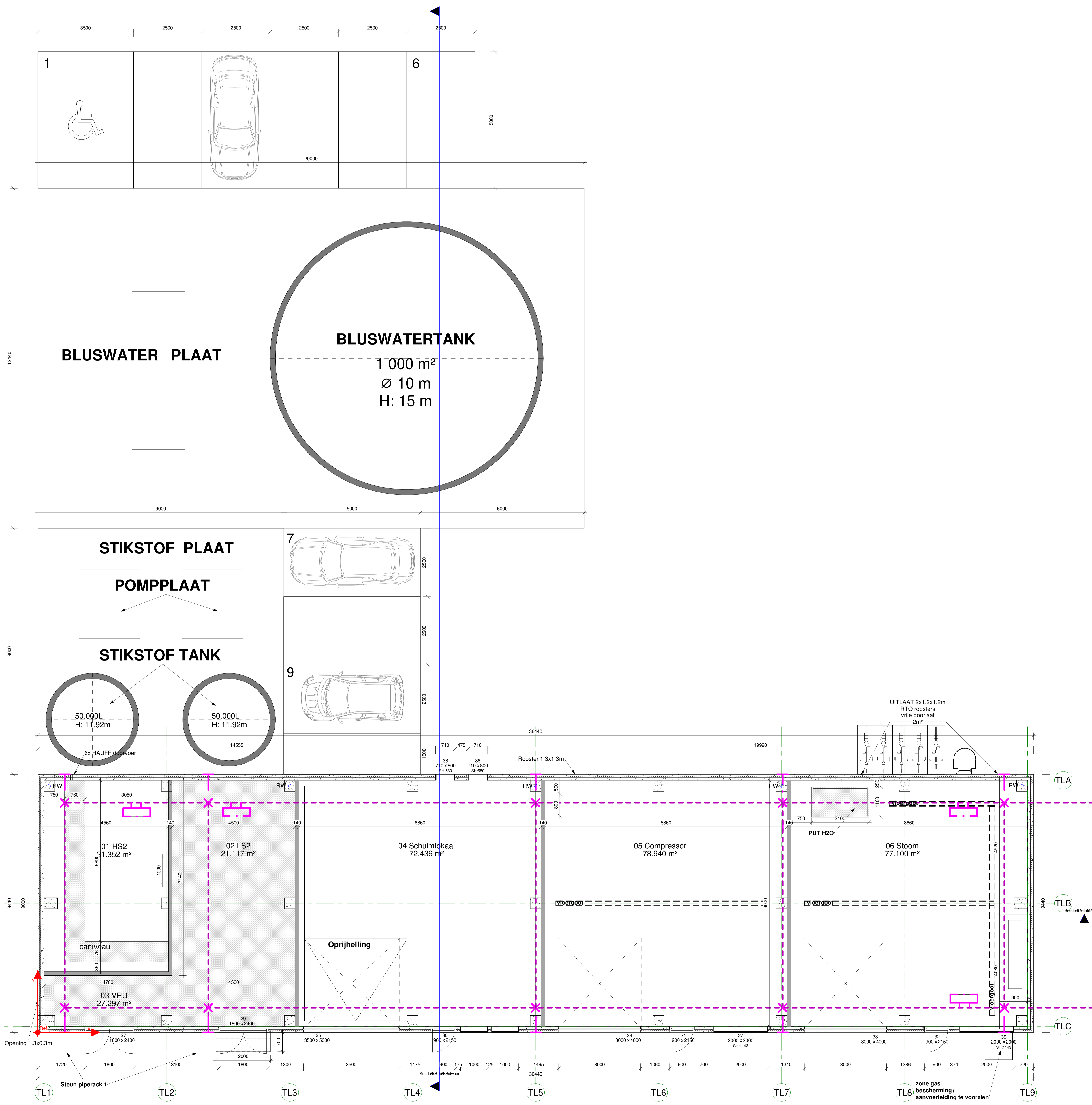
Gelijkvloers 1 : 50
