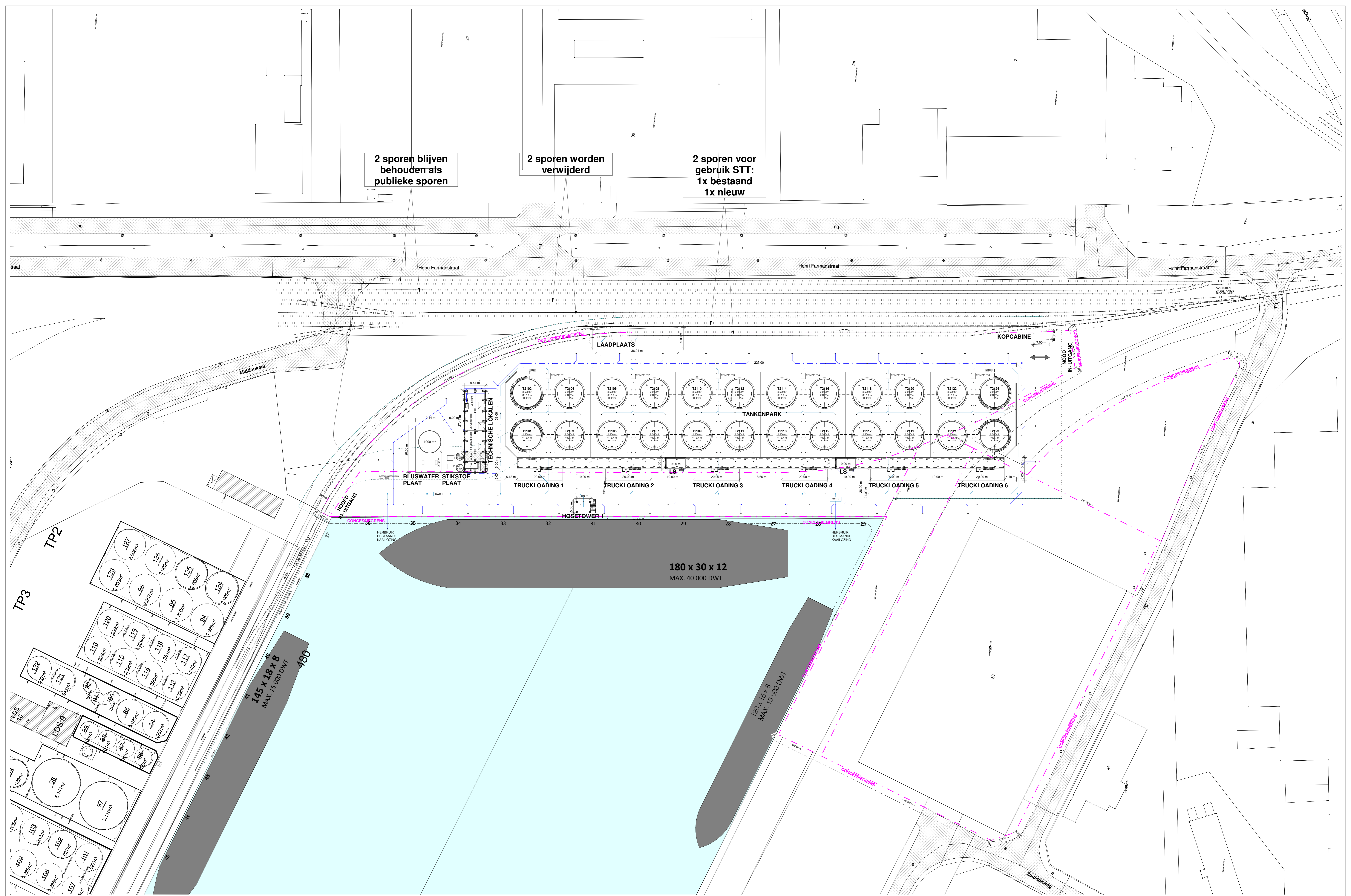
Algemene funderings- en roteringsplan 1 : 500
