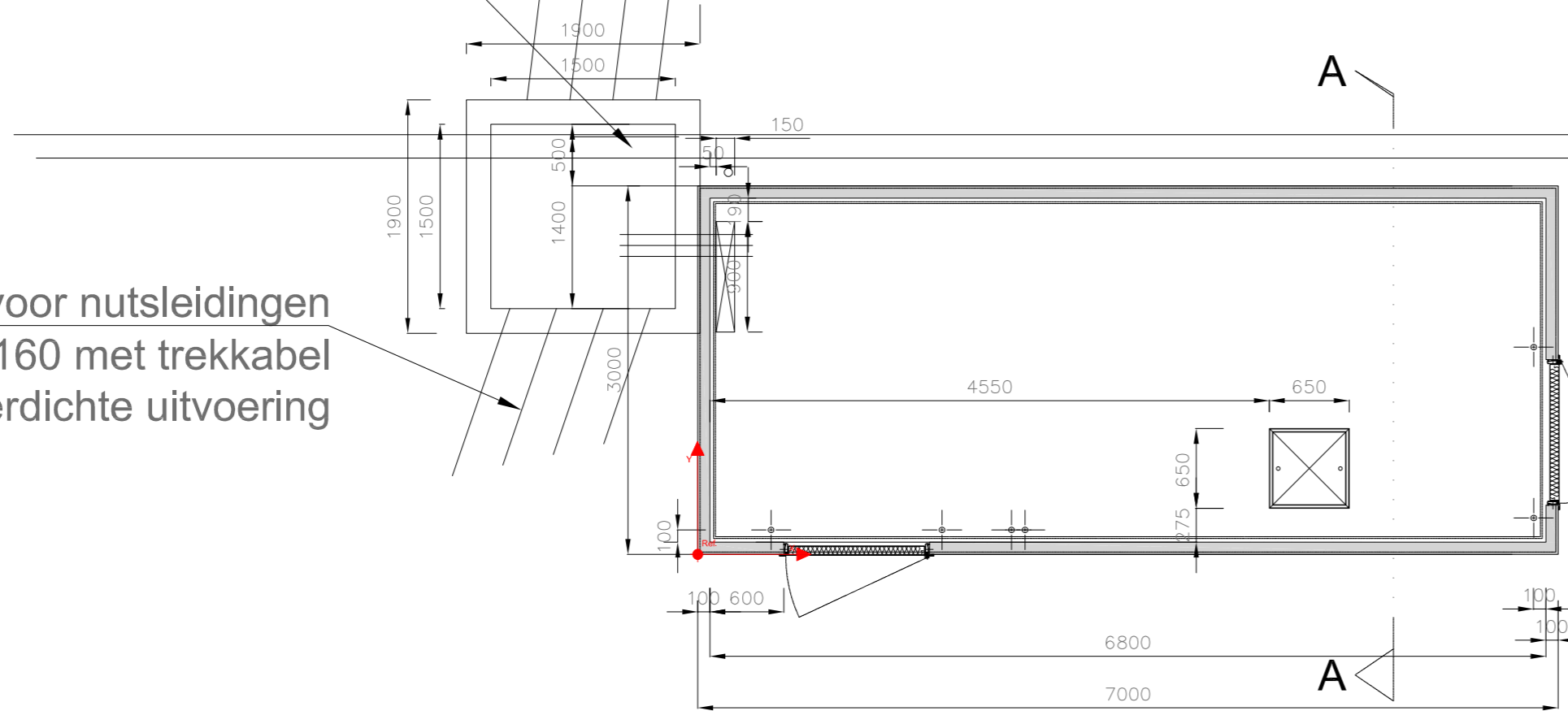
GRONDPLAN
