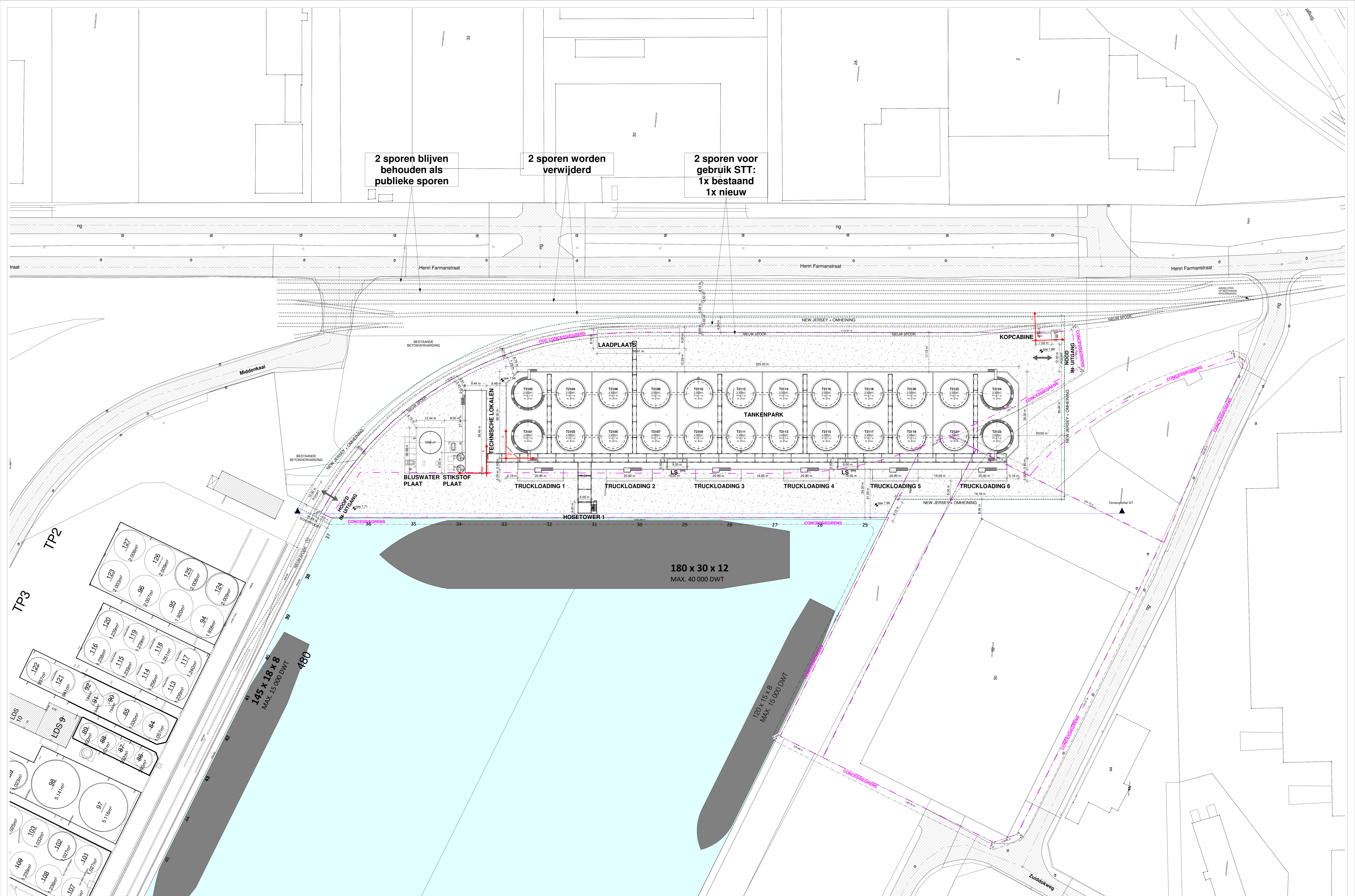
Inplantingsplan VT 1 : 500
