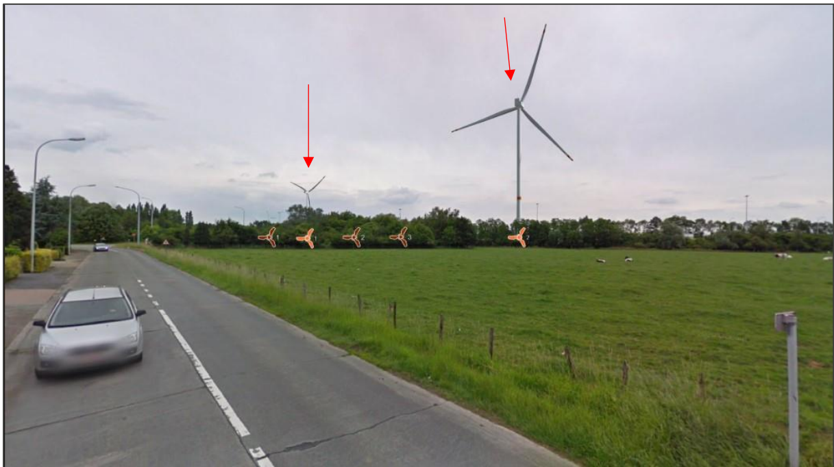
Figuur 56: Visualisatiepunt 4 – Groenstraat: nieuwe situatie met de nieuwe/geplande turbines
