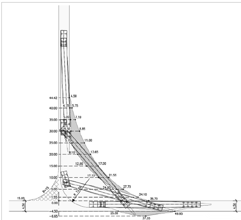
Figuur 32 : Voorbeeld verharding toegangsweg in bochten
