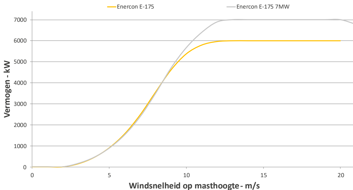
Figuur 11: Powercurves van eenzelfde windturbintype met een verschillend maximaal vermogen
