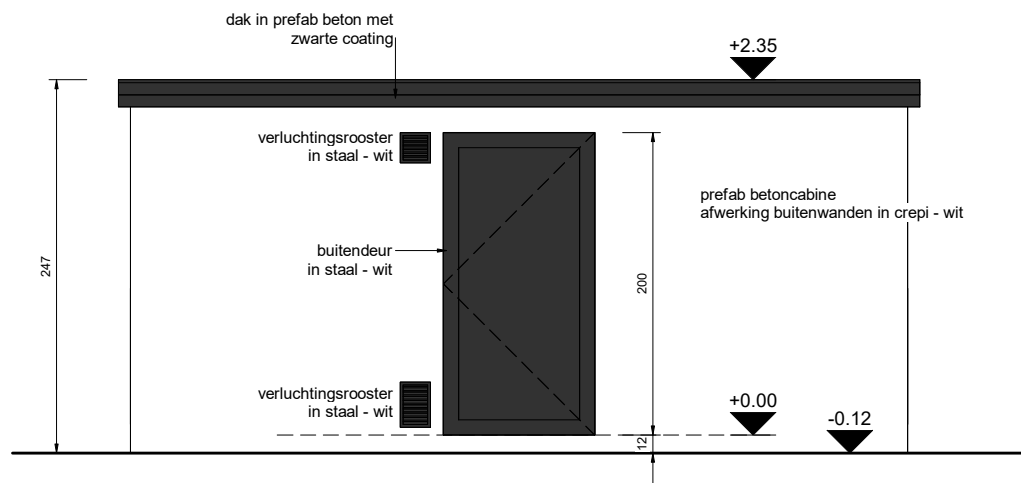
3 Vooraanzicht 1 : 50
