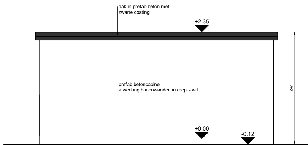
5 Achteraanzicht 1 : 50
