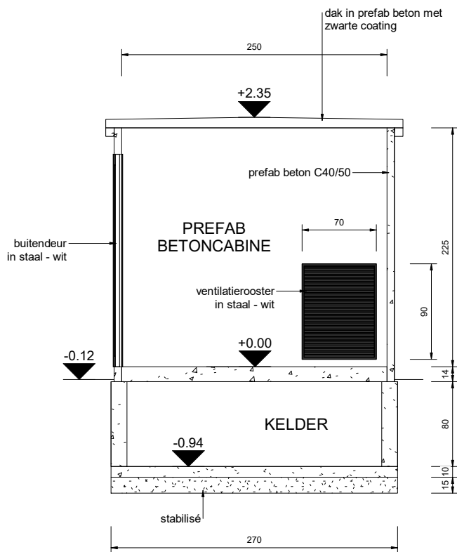
2 Dwarsdoorsnede 1 : 50
