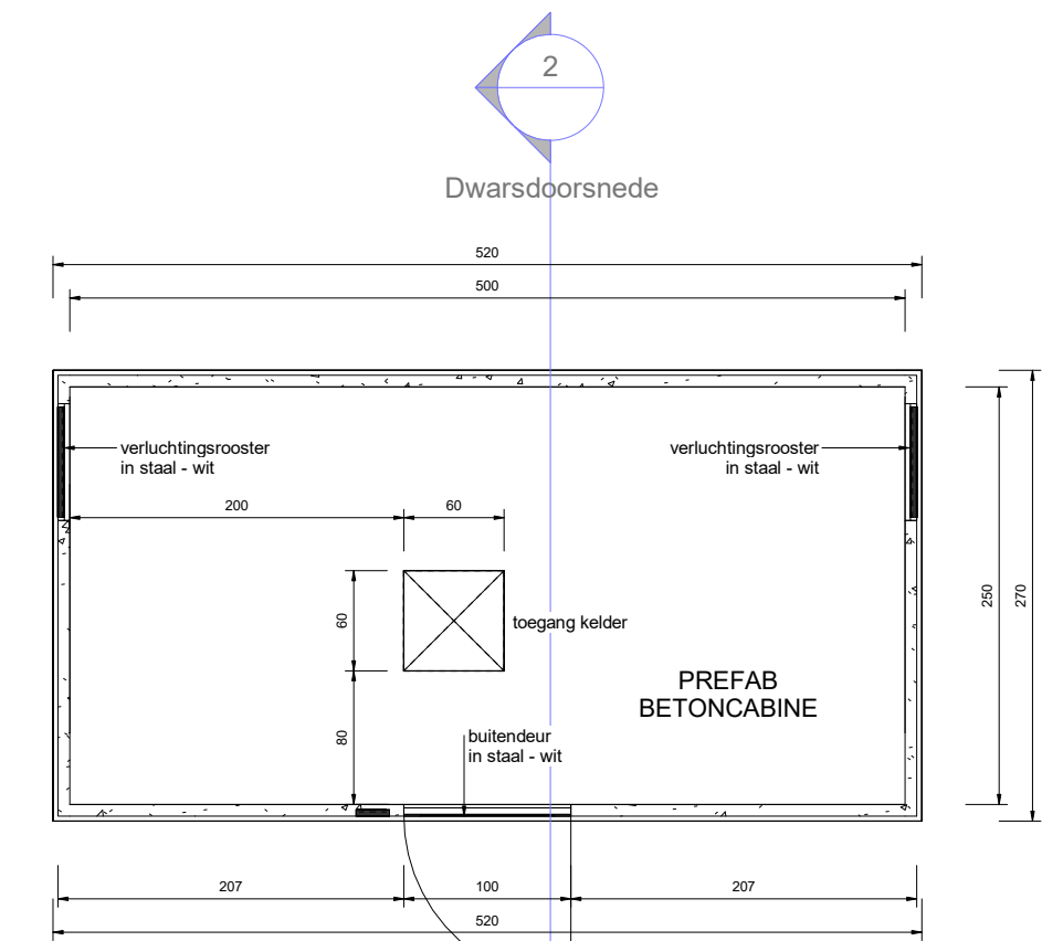
1 Grondplan 1 : 50
