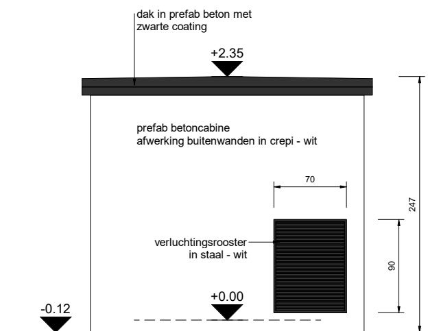
4 Linkerzijaanzicht 1 : 50
