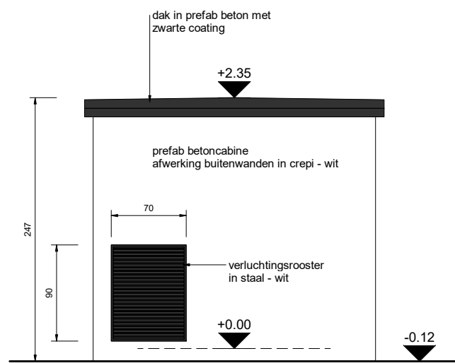
6 Rechterzijaanzicht 1 : 50
