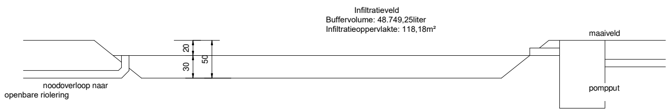
1 Infiltratieveld principesnede 1 : 50 0 0,5 1 1,5 2 2,5m
