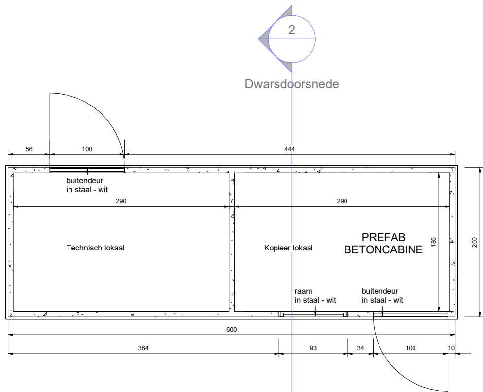
1 Grondplan 1 : 50
