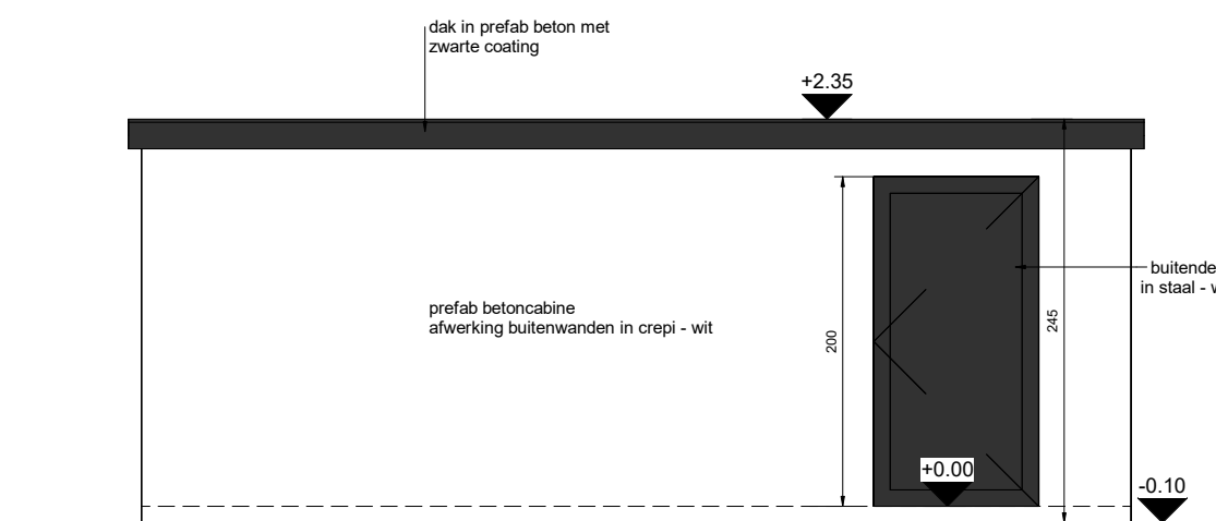
5 Achteraanzicht 1 : 50
