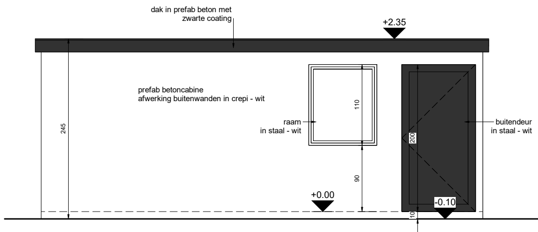
3 Vooraanzicht 1 : 50
