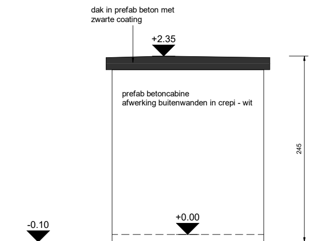
4 Linkerzijaanzicht 1 : 50
