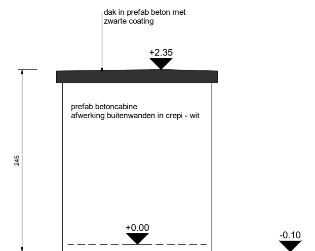
6 Rechterzijaanzicht 1 : 50
