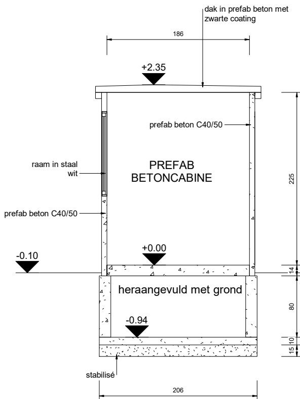
2 Dwarsdoorsnede 1 : 50
