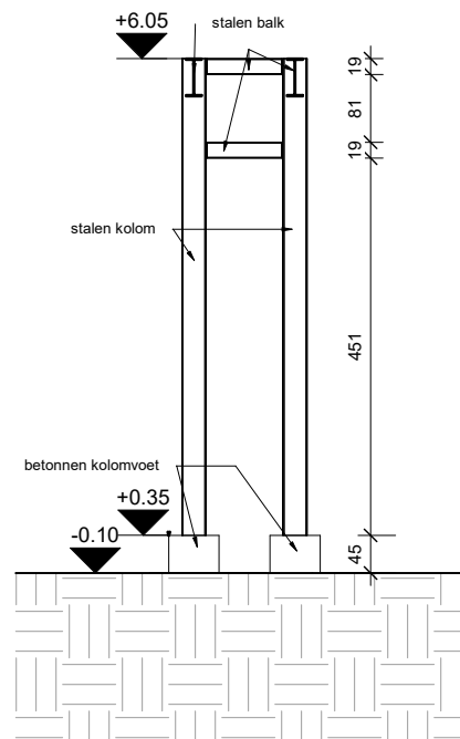
2 Leidingbrug B 1 : 100
