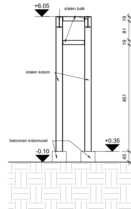
3 Leidingbrug C 1 : 100
