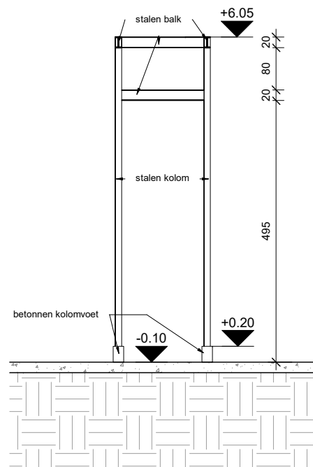
1 Leidingbrug A 1 : 100
