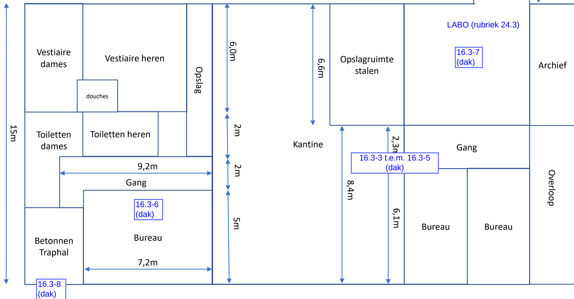
BIJLAGE C8A_3_Verdiepingsplan productiegebouw
