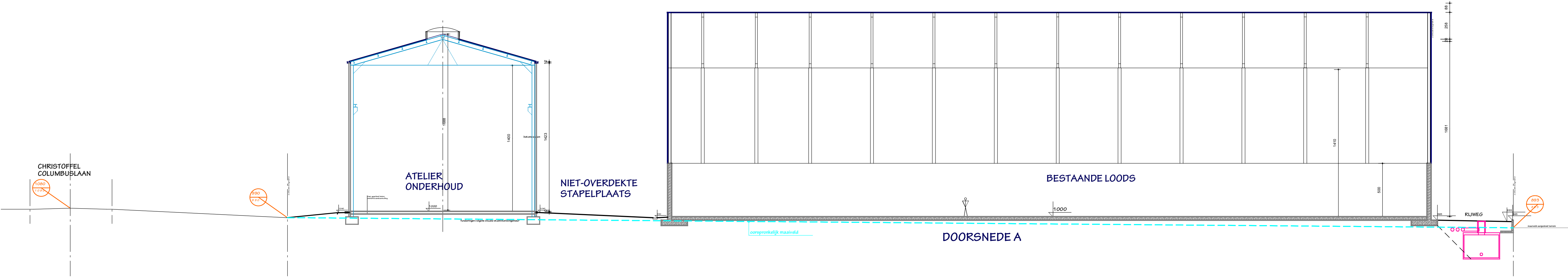
TERREINPROFIEL
