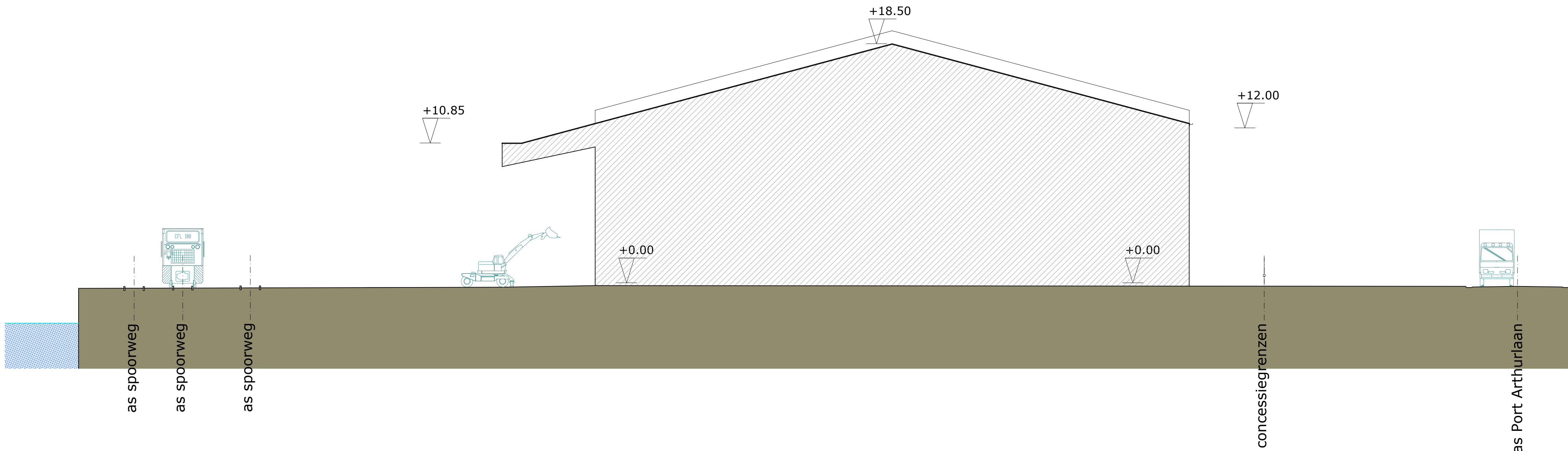
TERREIN PROFIEL NIEUW schaal: 1/200
