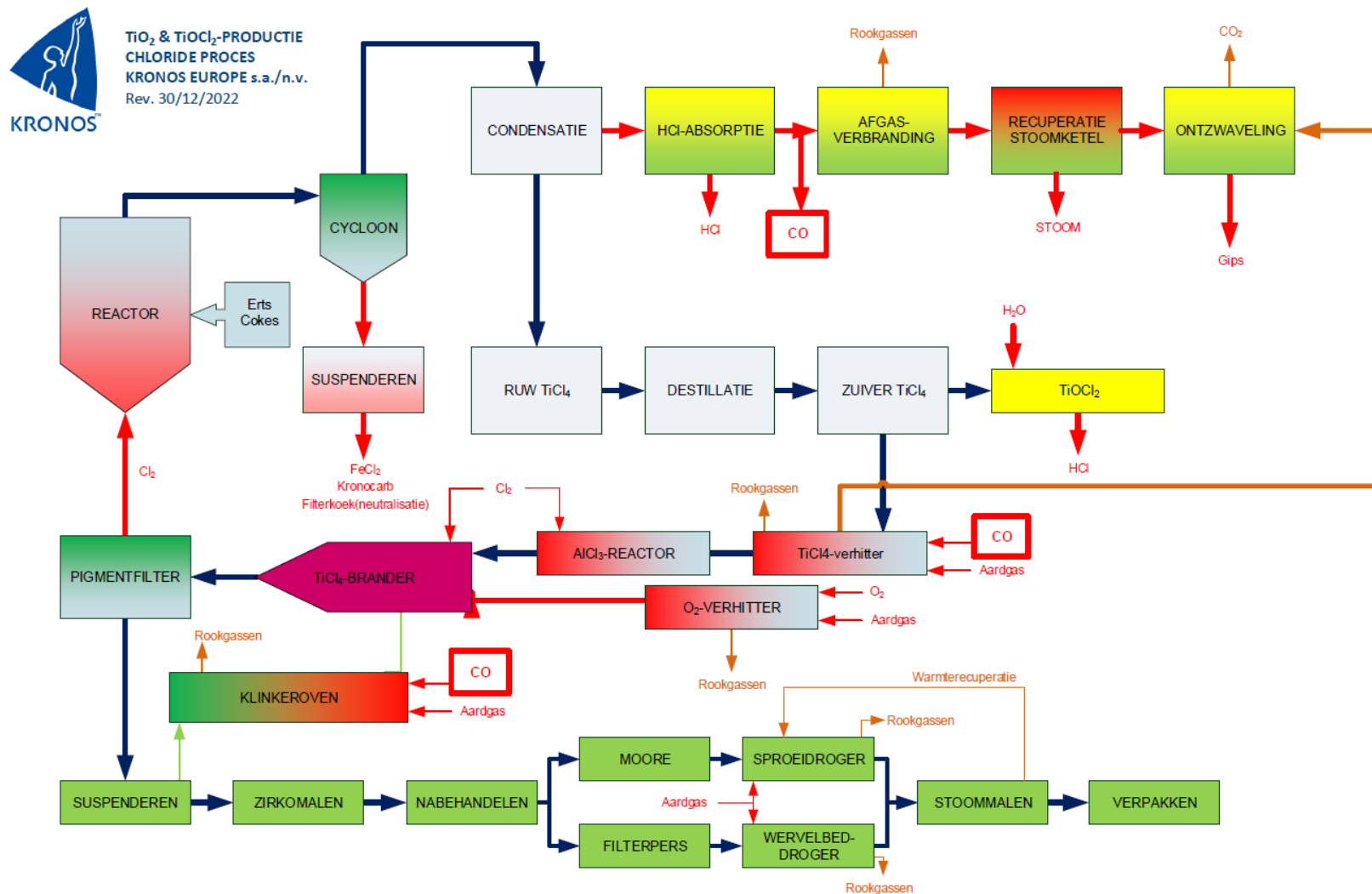
FIGUUR 1.10 BLOKSCHHEMA VAN HET PRODUCTIEPROCES. HET PRODUCTIEPROCES START IN DE WERVELBEDREACTOR
