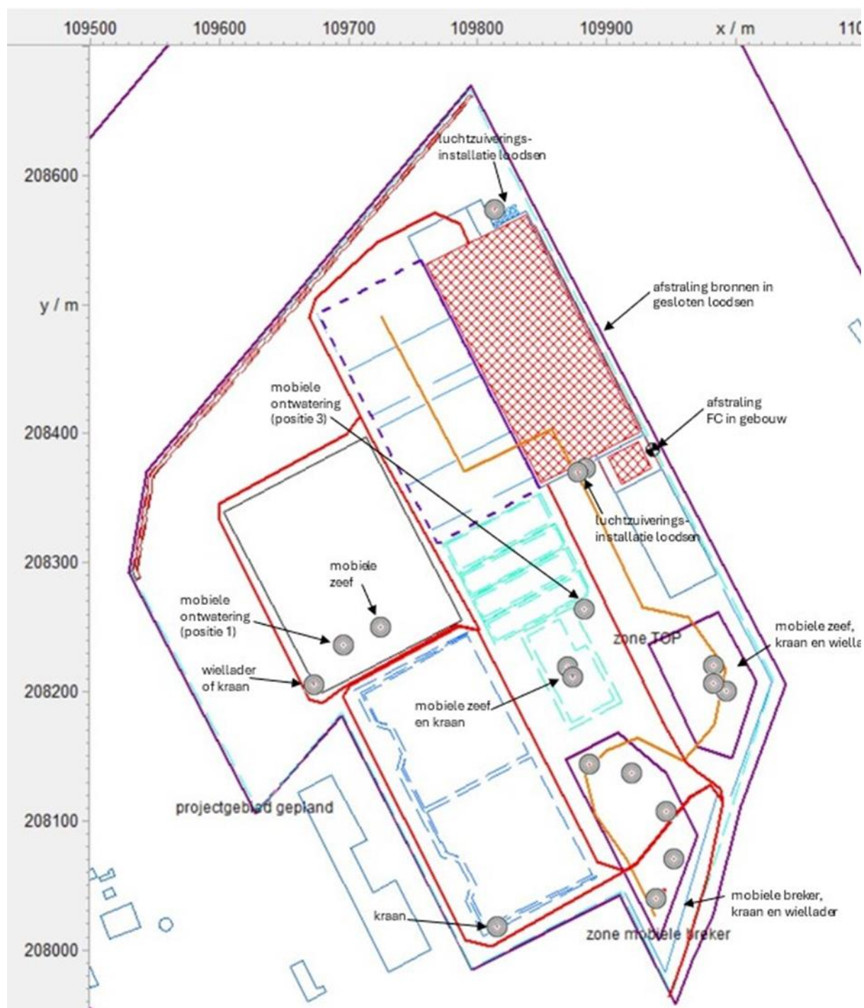
Figuur XII-8: Aanduiding geluidsbronnen in geluidsmodel, geplande situatie
