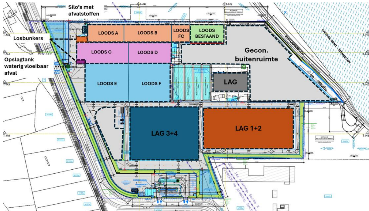
Figuur III-1: Inrichtingsplan terrein met aanduiding verschillende zones voor opslag en verwerking van afvalstoffen
