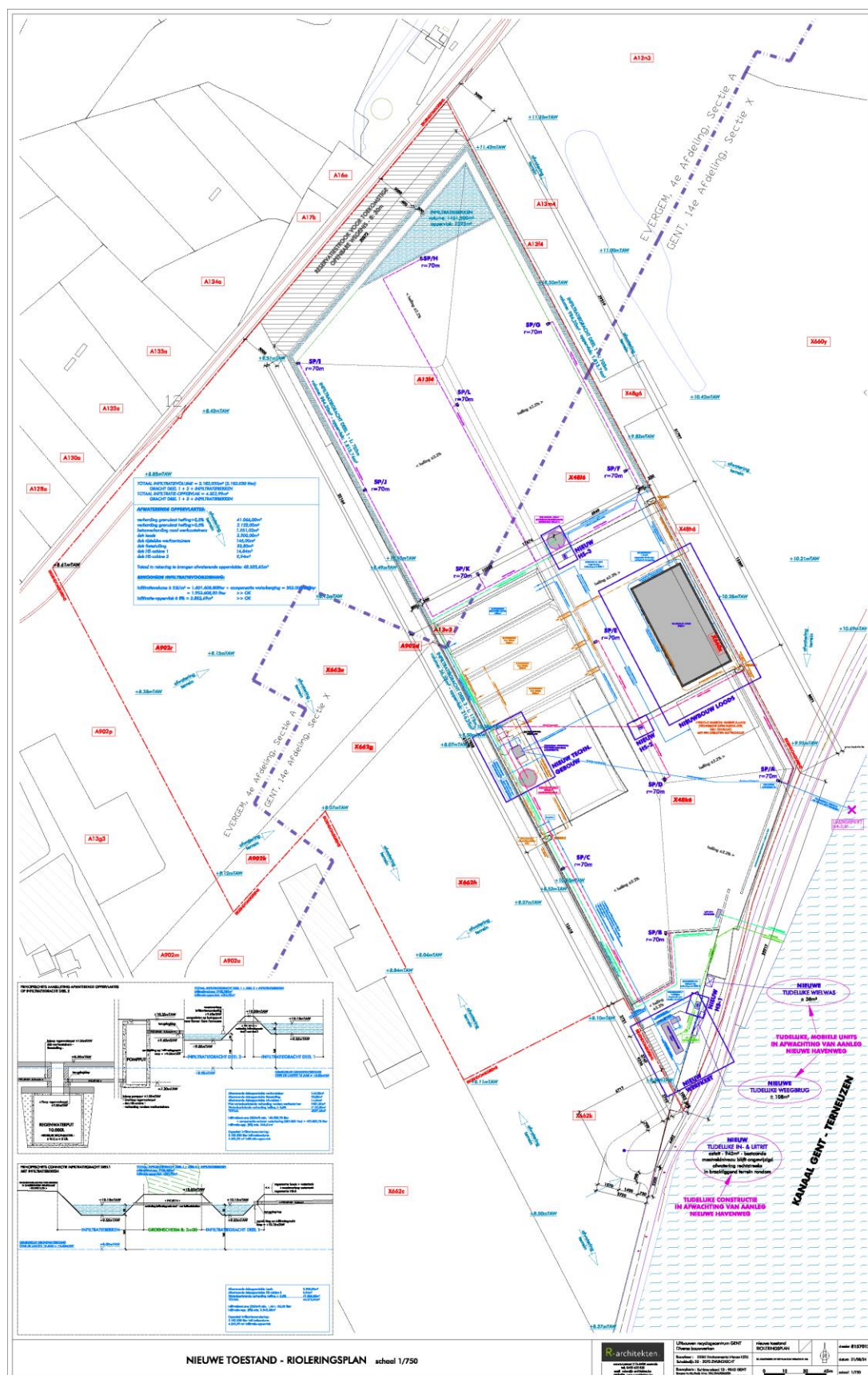
Figuur X-11: Algemeen overzicht van de referentiesituatie met de gehele projectsite rood omrand (bron: bedrijf)
