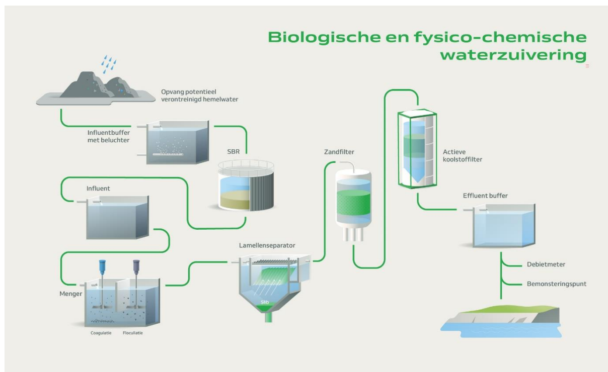
Figuur III-20: Schematische weergave uitgebreide configuratie waterzuivering (Bron: Initiatiefnemer)
