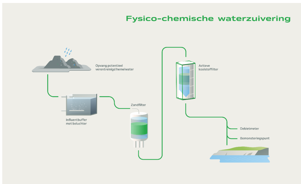
Figuur III-19: Schematische weergave standaardconfiguratie waterzuivering (Bron: Initiatiefnemer)
