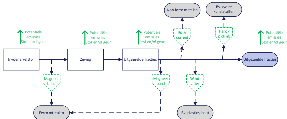
Figuur III-8: processchema mechanische behandeling d.m.v. zeven – met optionele zuiveringsstappen door magneetbanden, eddy current, windzifter en handpicking (Bron: Initiatiefnemer)
