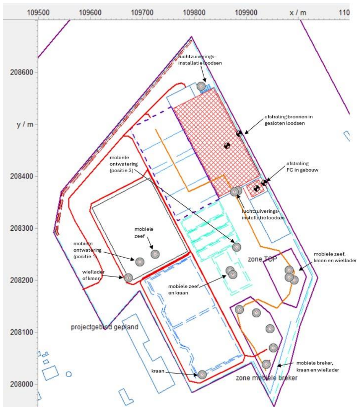
Figuur XII-9: Aanduiding geluidsbronnen in geluidsmodel, ontwikkelingsscenario
