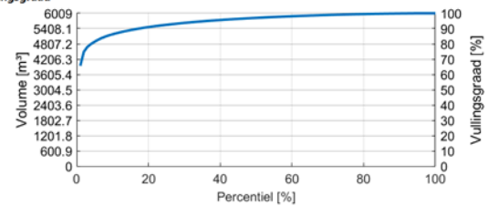
Figuur X-14: Siriomodellering regenwaterput - hergebruik niet-verontreinigd hemelwater
