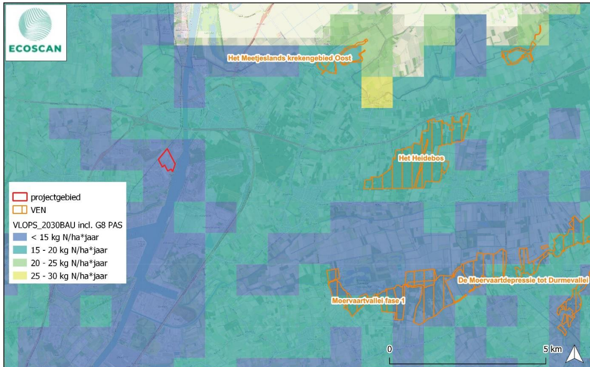
Figuur XIII-23: Vermestende deposities ter hoogte van de dichtstbijgelegen VEN-gebieden o.b.v. VLOPS BAU 2030 (incl. reductiemaatregelen)
