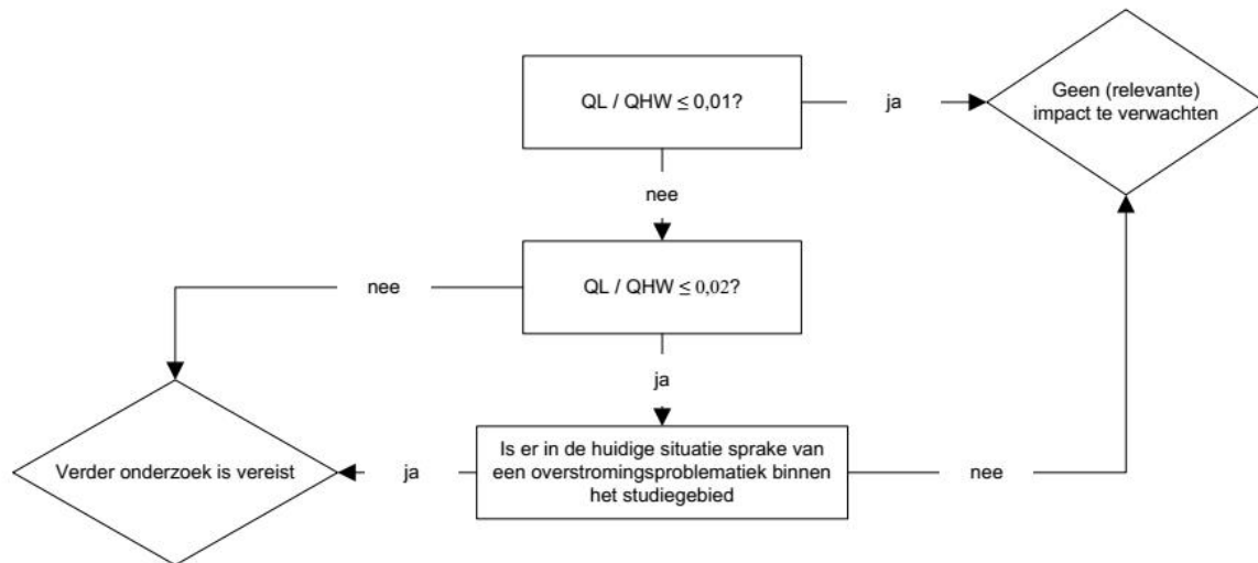
Figuur X-10: Beoordelingskader hydraulische impact oppervlaktewaterlozing
