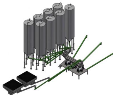
Figuur III-17: Visuele weergave vaste batchinstallatie (Bron: Initiatiefnemer)
