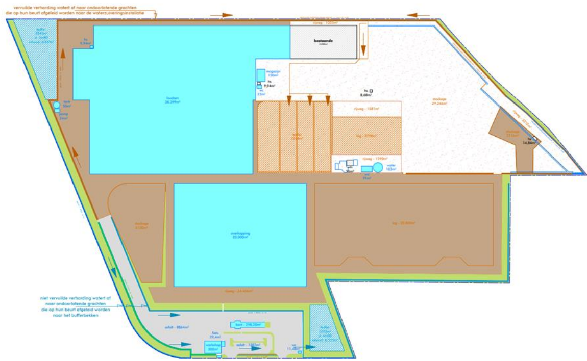
Figuur X-13: Algemeen overzicht van het projectgebied in de geplande situatie
