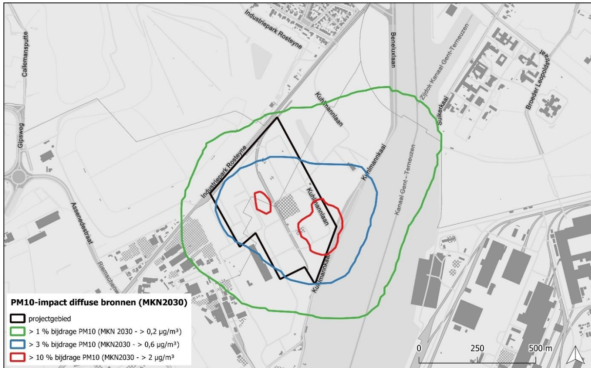
Figuur IX-9: Stofimpact PM 10 gewenste situatie bij MKN 2030
