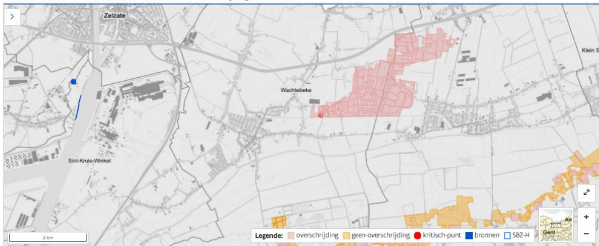
Figuur XIII-20: Output Impactscore voor de exploitatiefase (stationaire bronnen en verkeer) – geplande situatie
