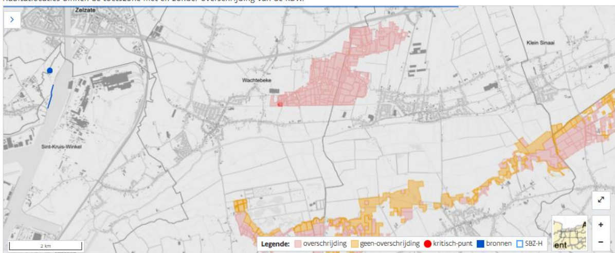
Figuur XIII-16: Output Impactscore voor de exploitatiefase (stationaire bronnen en verkeer) – huidig vergunde situatie
