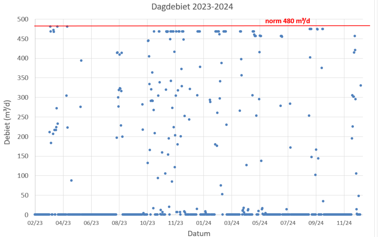
Figuur X-12: Overzicht lozingsdebieten 2023-2024 (dagbasis)
