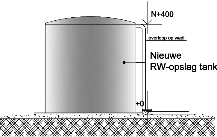
Aanzicht -1/100-
