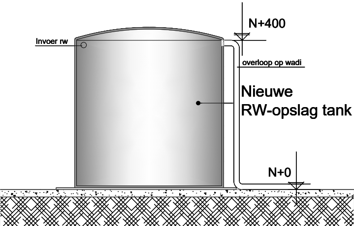
Snede -1/100-
