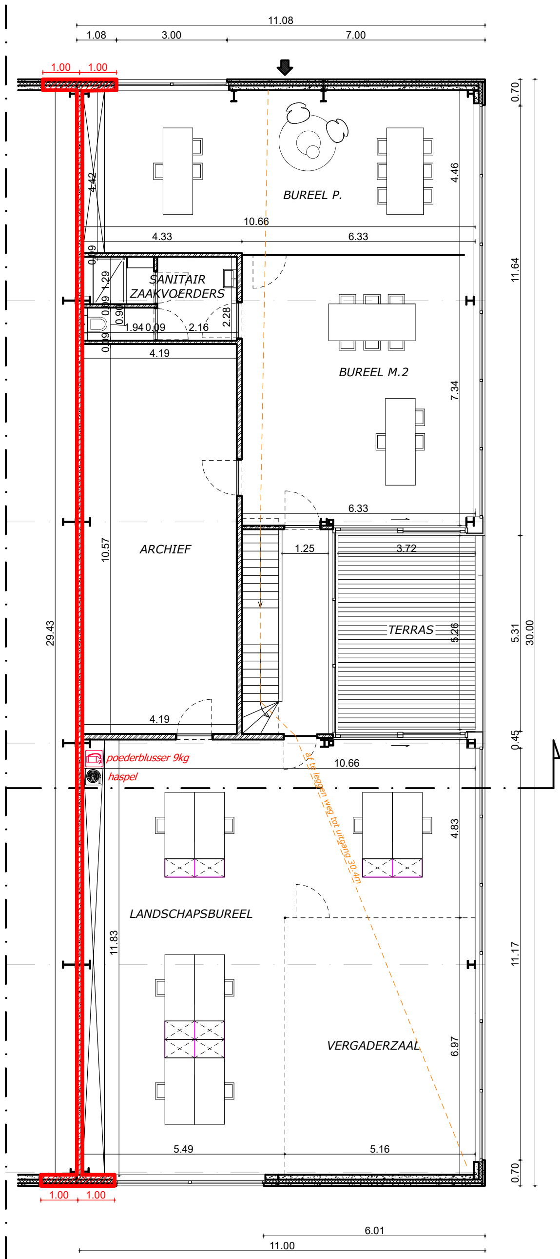
VERDIEPINGSPLAN 1 BLOK 7 wijziging reeds vergunde plannen
