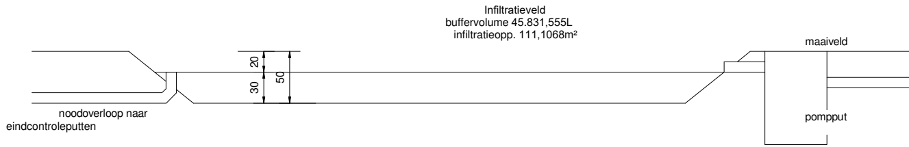
1 Infiltratieveld principesnede 1 : 50 0 0,5 1 1,5 2 2,5m
