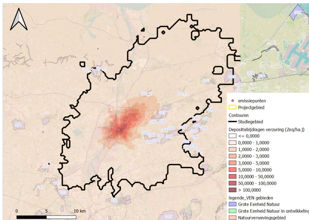
Figuur 3: Depositiecontour verzurende deposities (Zeq/ha.j)
