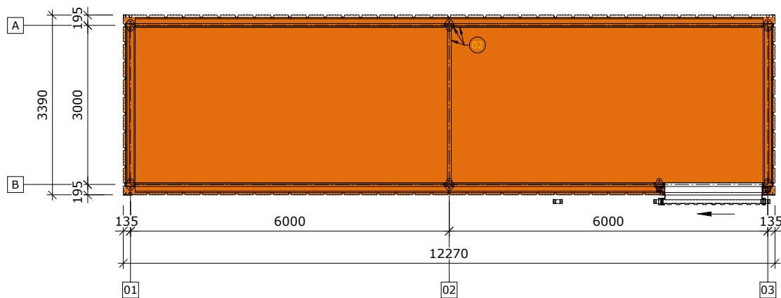
GROND PLAN
