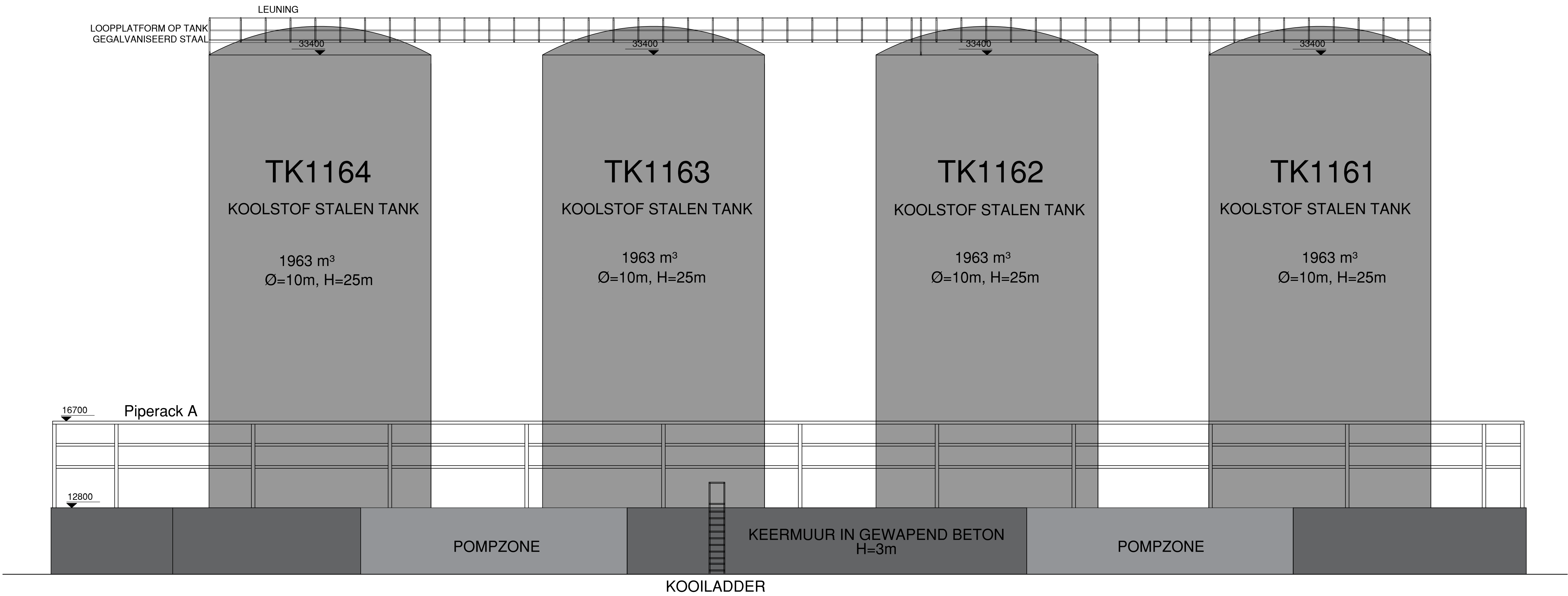
Aanzicht oost
