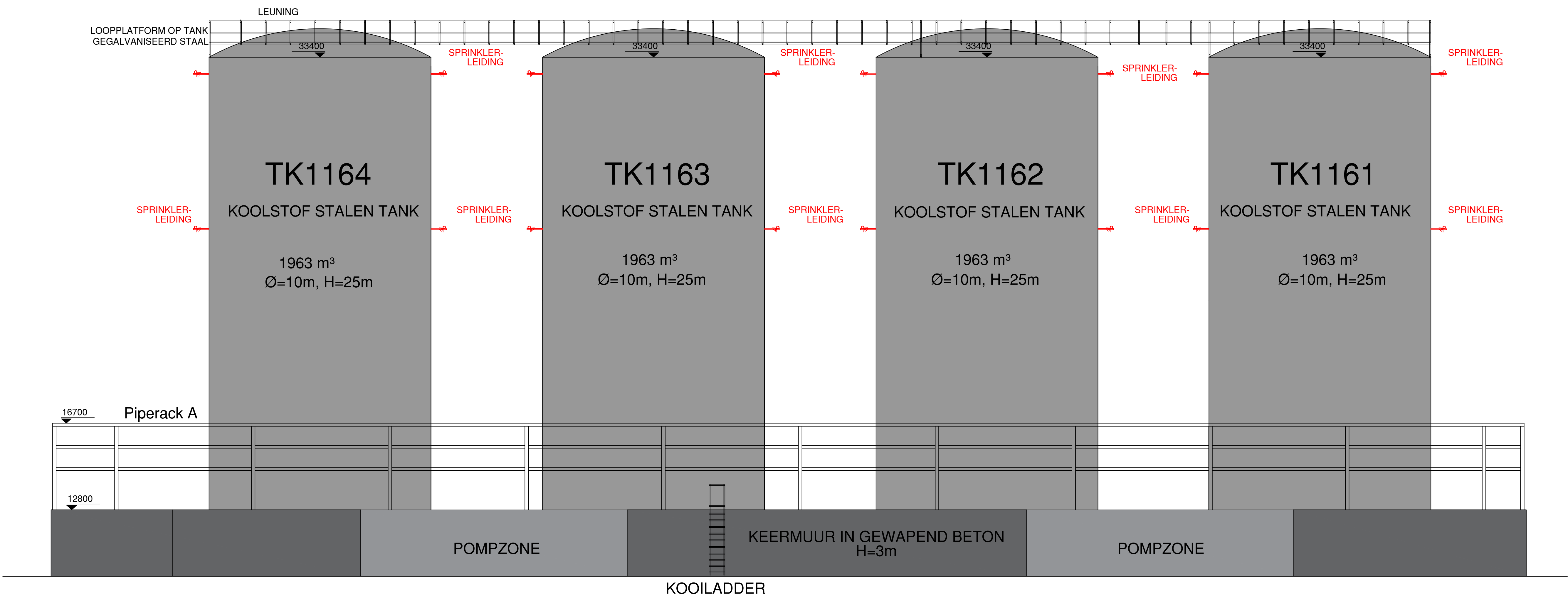
Aanzicht oost
