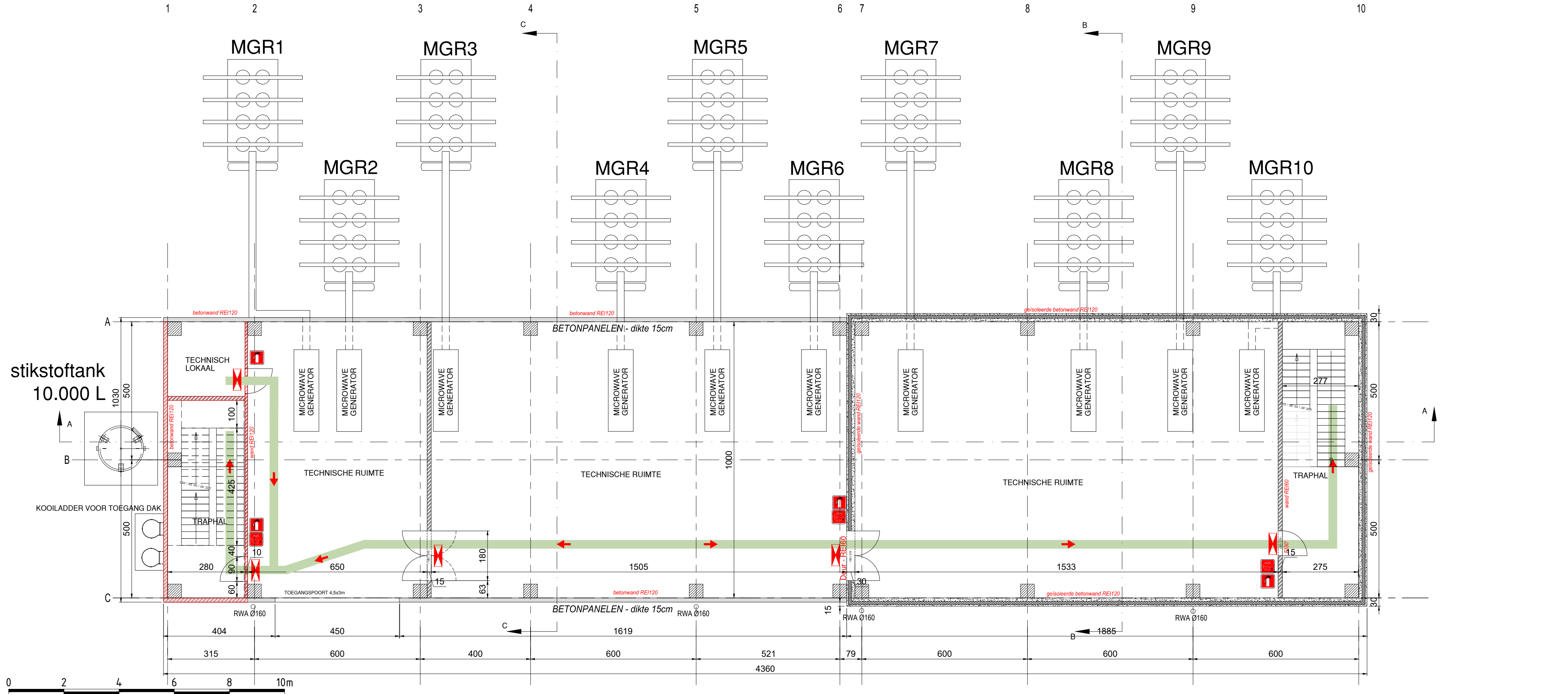
schaal: 1/100 BA_OPERATIONEEL GEBOUW_PB_N_02_NIVEAU +01
