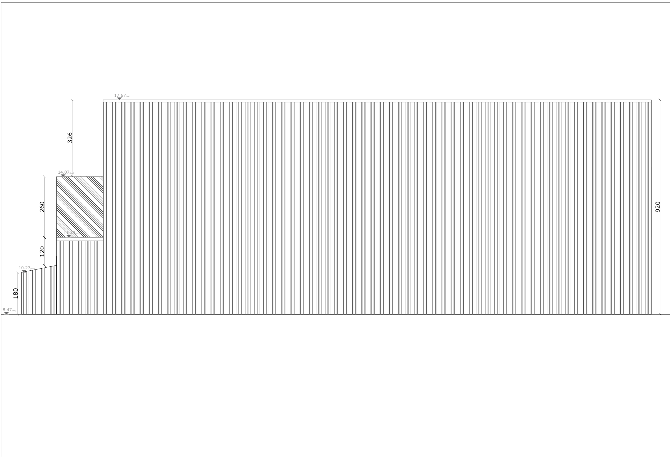
Gevelaanzicht noord- vergunde toestand 'SH2 loods' - 1/100
