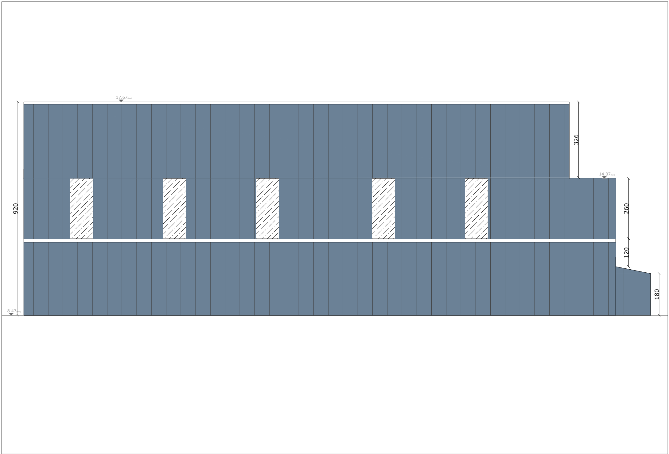
Gevelaanzicht zuid - bestaande toestand 'SH2 loads' - 1/100
