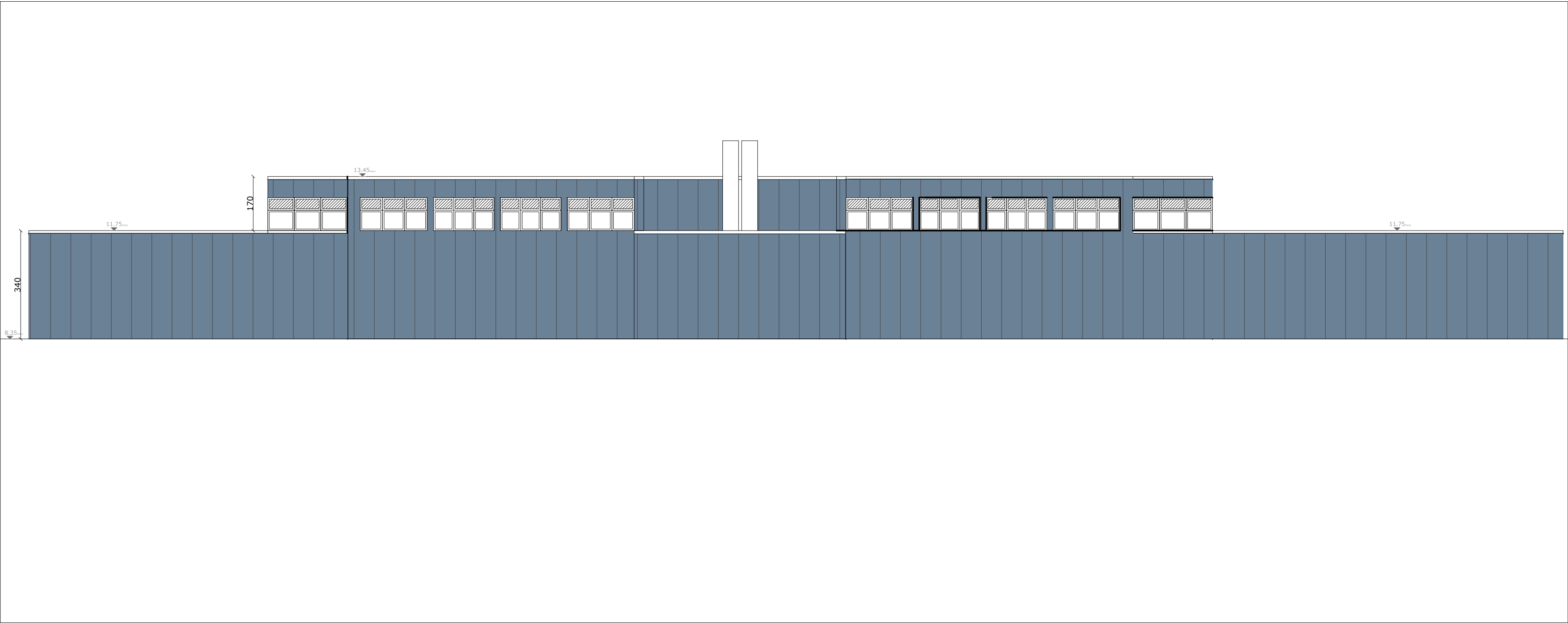
Gevelaanzicht west - bestaande toestand 'SH1 kantoren' - 1/100
