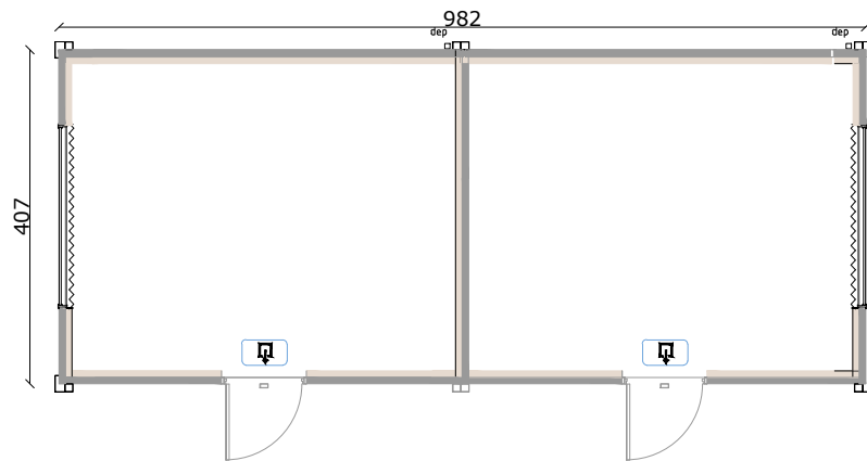
Grondplan
