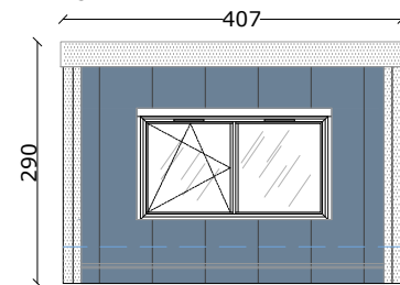
zijkantaanzicht
