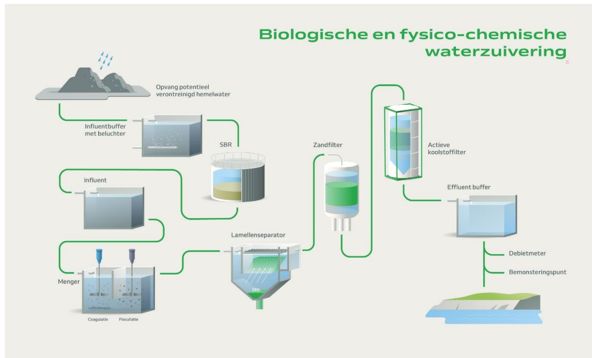
Figuur 2: Schematische weergave uitgebreide configuratie waterzuivering
