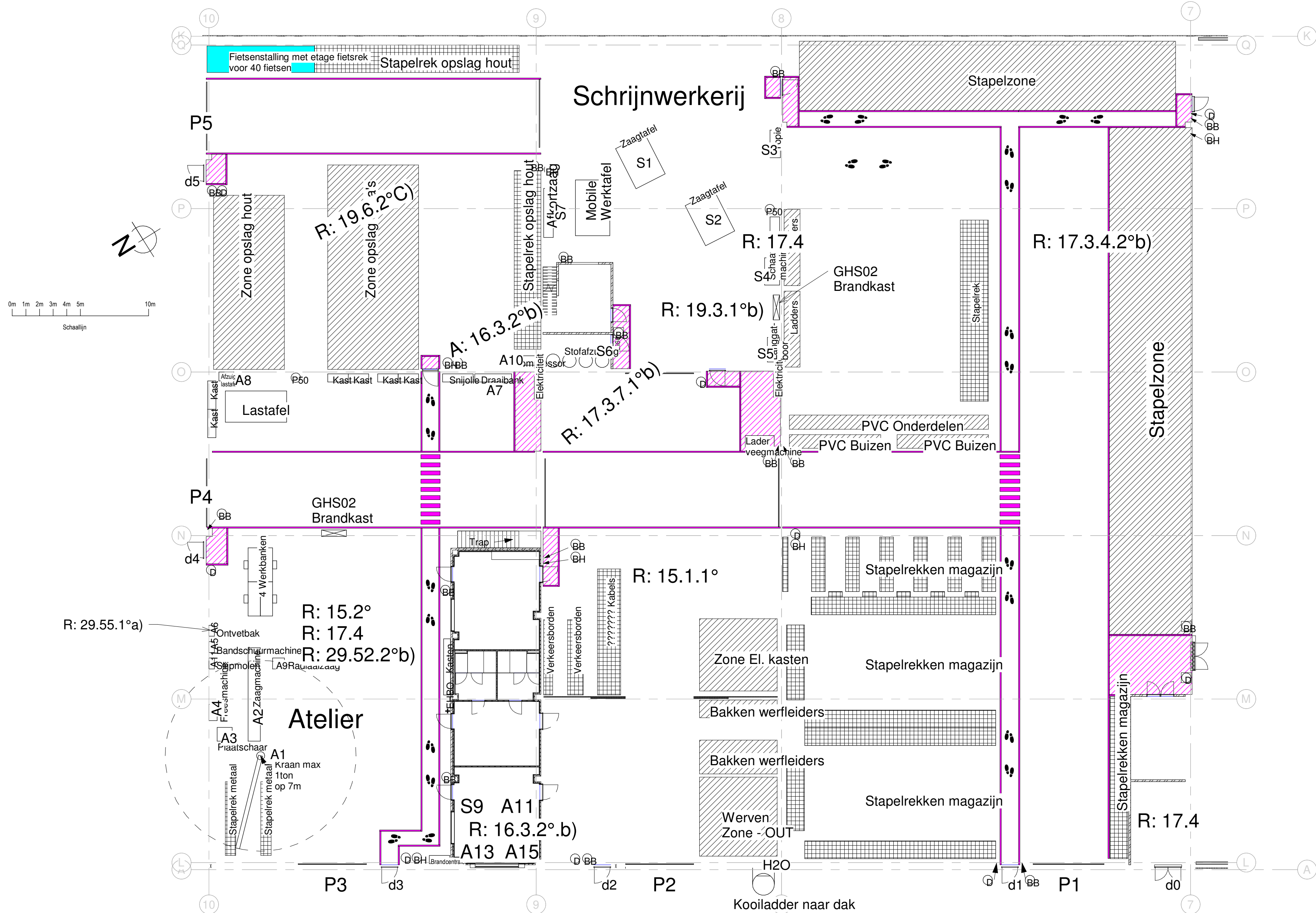
UITRUSTING LOODS. Schaal 1/200
